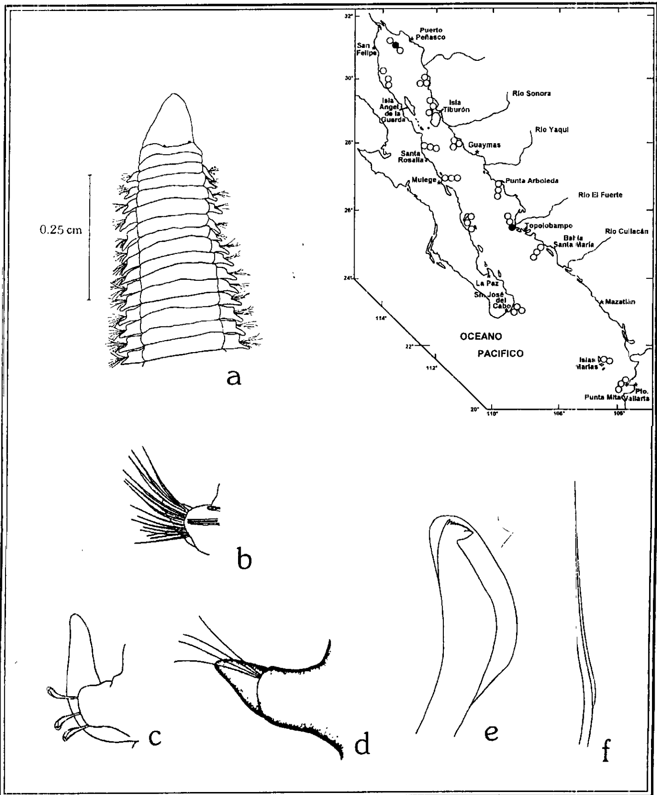
Figura 19.7: Lumbrineris erecta : a) Región anterior, vista dorsal; b) Parapodio anterior; c) Parapodio posterior con lóbulos postsetales elongados; d) Parapodio 5; e) Gancho cubierto del setígero posterior; f) Seta limbada. Figs. b, c, f: tomadas de Moore 1904; Figs. d, e: tomadas de Fauchald 1970.
