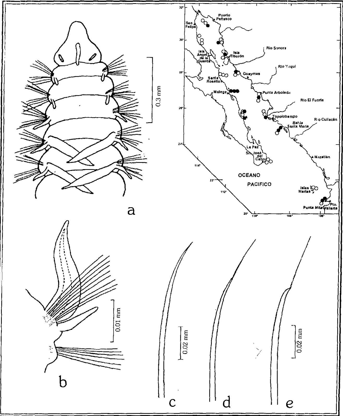
Figura 23.6. Aricidea (Allia) suecica : a) Región anterior, vista dorsal; b) Parapodio del setígero 7; c) Neuroseta modificada del setígero 28; d) Neuroseta modificada del setígero 36; e) Neuroseta modificada del setígero 55. Figs. Tomadas de Gaston 1984.
