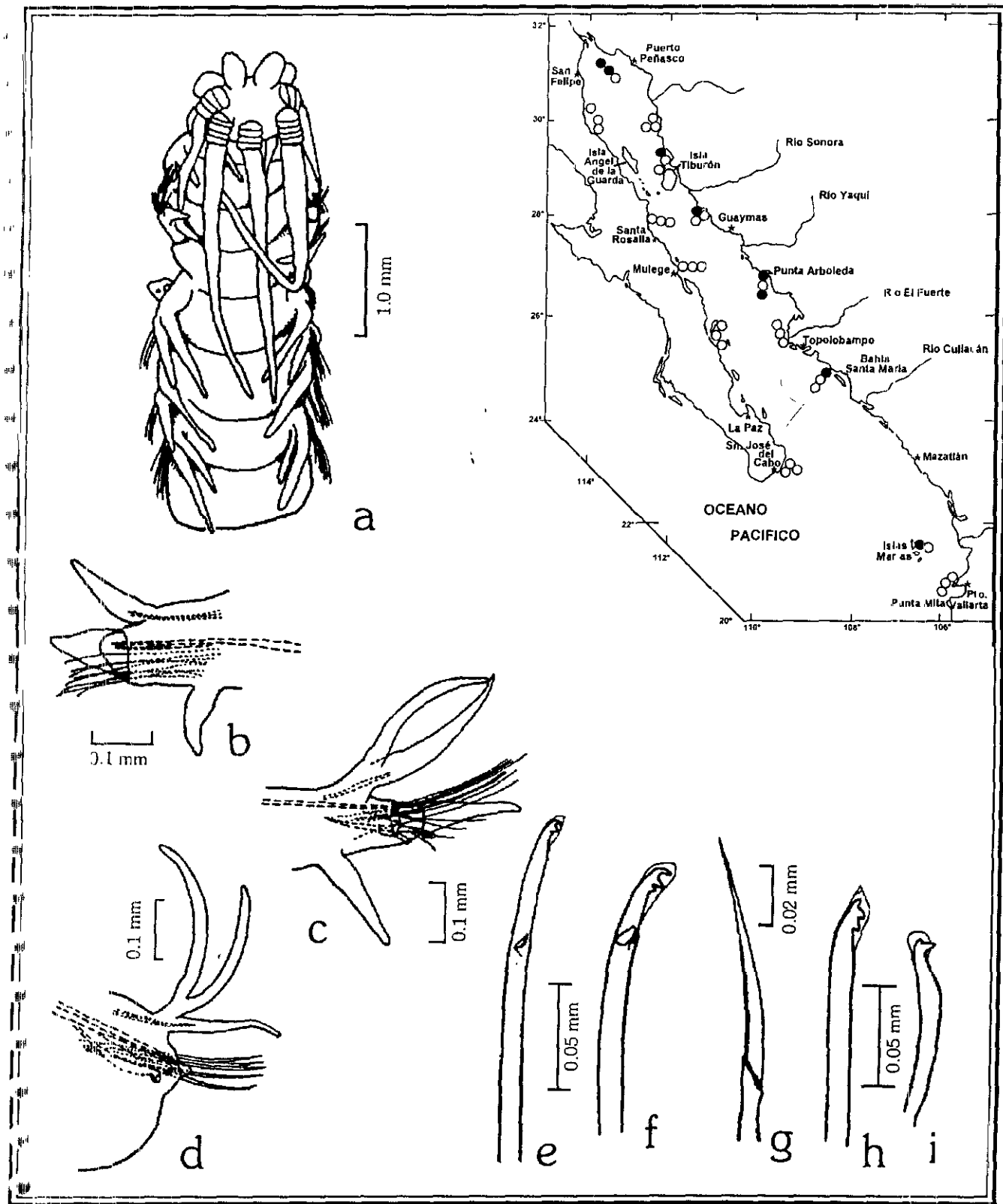
Figura 17.16. Mooreonuphis nebulosa : a) Región anterior, vista dorsal; b) Primer setígero; c) Setígero 6; d) Setígero 25; e) Seta pseudocompuesta superior; f) Seta pseudocompuesta central, larga; g) Espiniger compuesto; h) Gancho largo del setígero 6; i) Gancho subcircular. Figs. a-f, h i: tomadas de Gathof 1984; Fig. g: tomada de Hartman 1944d.
