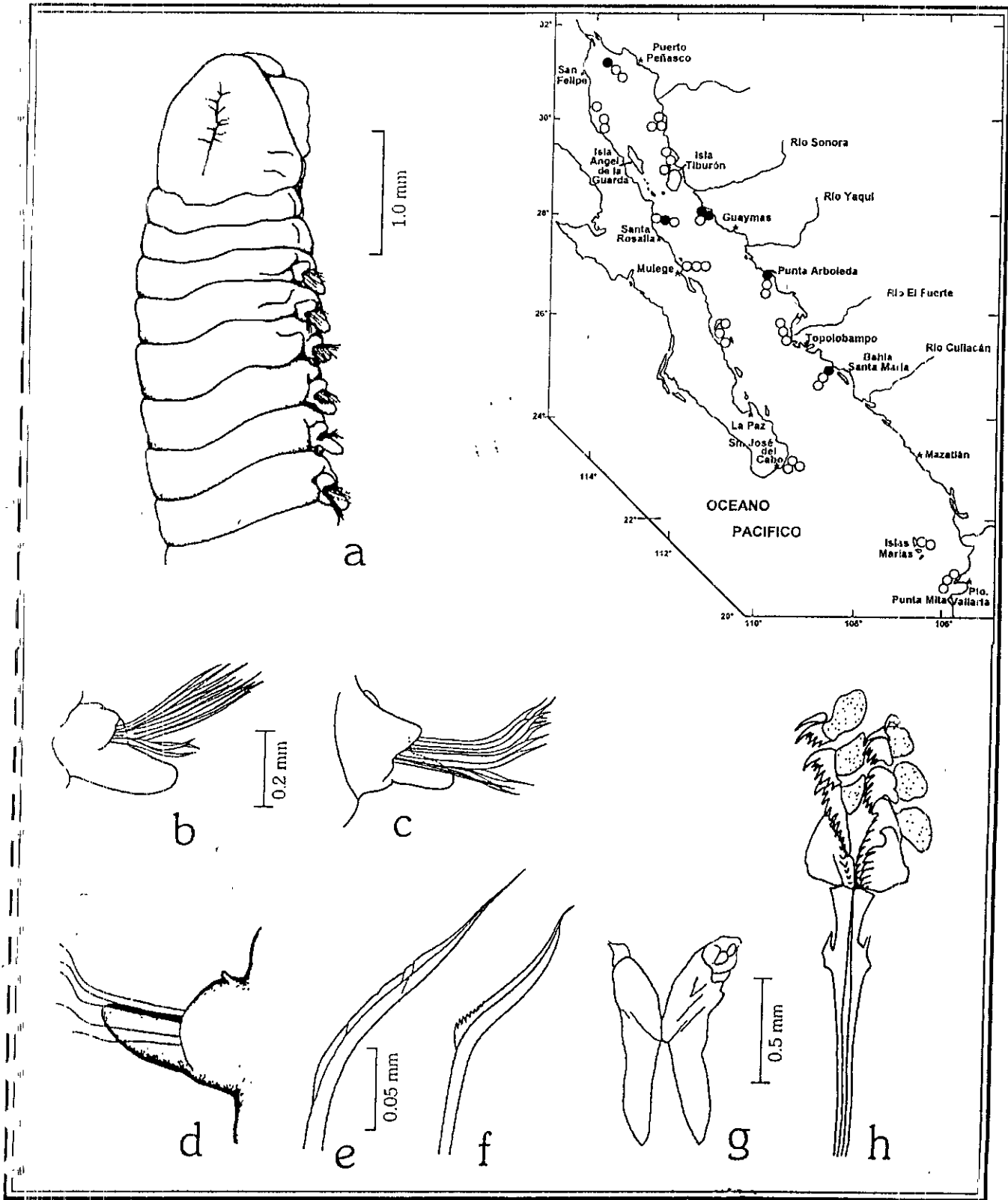
Figura 20.1 Arabella (Arabella) iricolor : a) Región anterior, vista ventral; b) Parapodio del setífero 8. c) Parapodio de la región media del cuerpo; d) Parapodio posterior; e) Seta limbada de la región media del cuerpo; f) Seta limbada, marginalmente aserrada; g) Maxilas; h) Mandibulas. Figs. a-c, g,h: tomadas de Uebelacker 1984; Fig. f: tomada de Fauvel 1923; Fig. d: tomada de Fauchald 1970.
