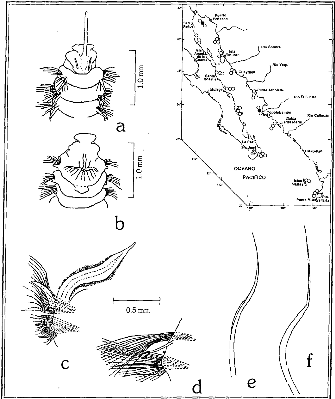
Figura 23.5. Aricidea (Aedicira) pacifica : a) Región anterior, vista dorsal; b) Región anterior, vista ventral; c) Parapodio del segmento 10; d) Parapodio posterior; e, f) Notosetas modificadas, con arista distal. Figs. a-d: tomadas de Strelzov 1979; Figs. e, f: tomadas de Hartman 1969.
