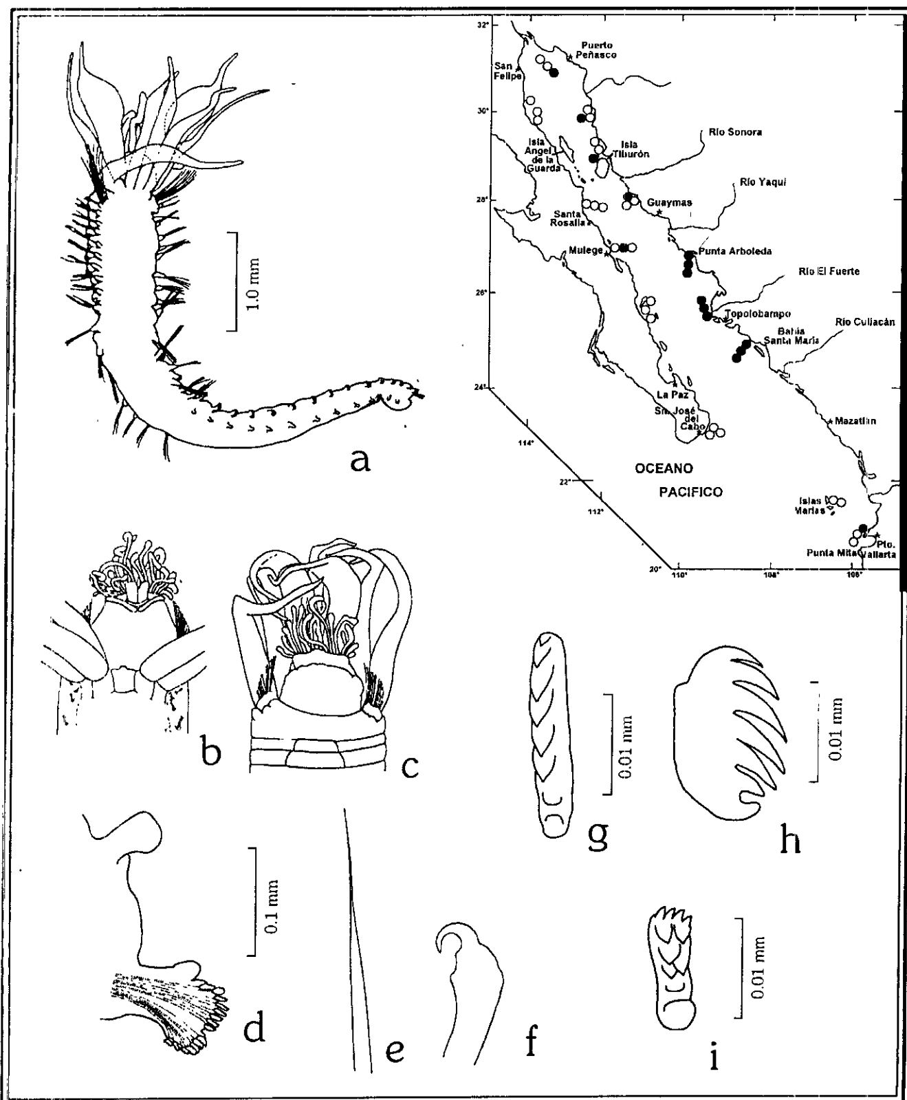
Figura 37.1. Amphicteis scaphobranchiata : a) Organismo completo; b) Prostomio; c) Tentáculos orales, d) Parapodio abdominal; e) Palea terminada en punto; f) Branquia foliosa con terminación en gancho; g) Uncino torácico; h) Uncino abdominal anterior; i) Uncino abdominal posterior. Figs. a, d, g-i: tomadas de Uebelacker 1984; Figs. b, c., e, f: tomadas de Moore 1906.
