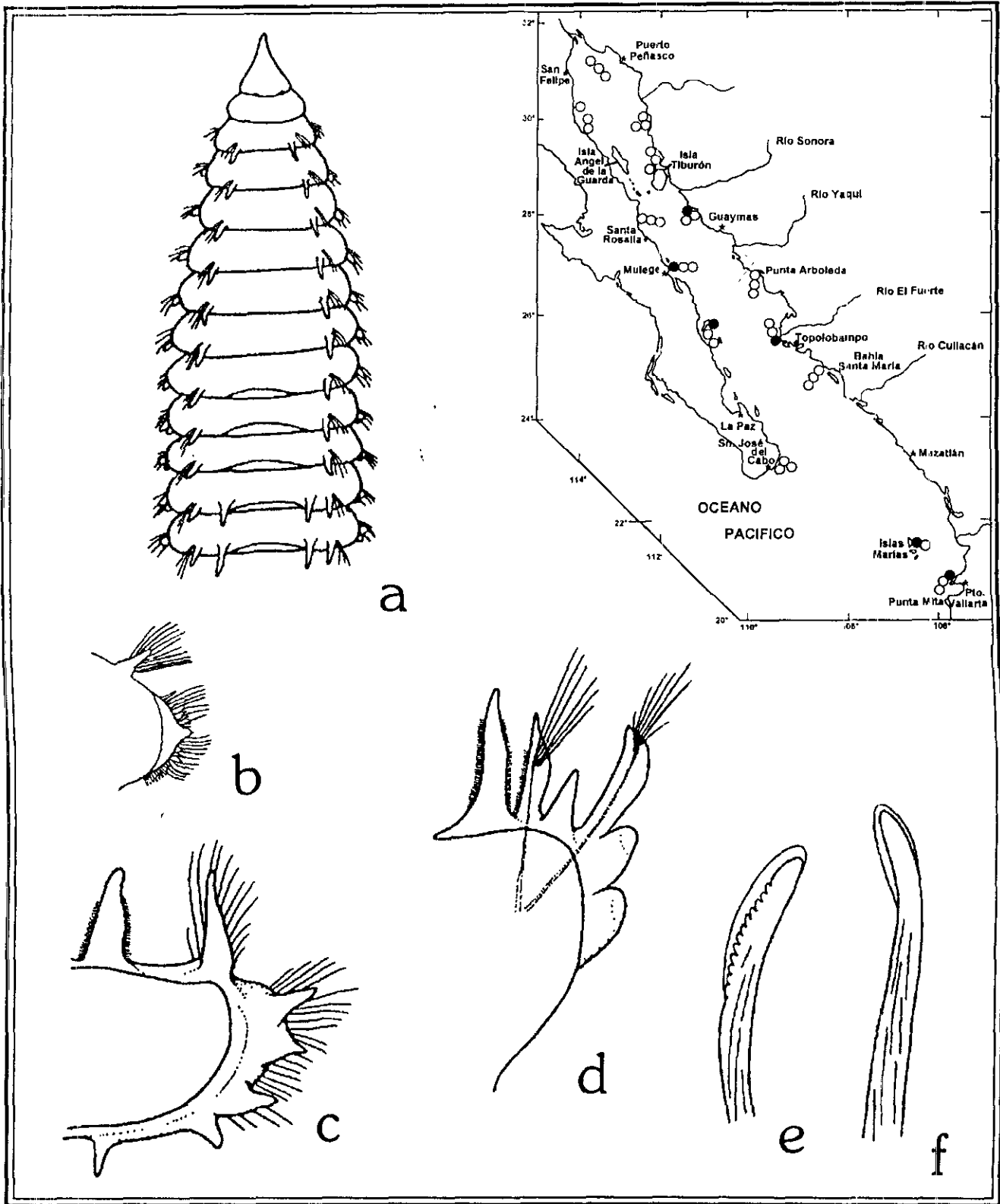
Figura 22.5. Orbinia riseri : a) Región anterior, vista dorsal; b) Sexto setígero; c) Décimo octavo parapodio torácico; d) Parapodio abdominal posterior; e) Espina neuropodial torácica; f) Espina neuropodial abdominal. Figs. a, c-e: tomadas de Day 1973; Fig. b: tomada de Pettibone 1963a; Fig. f: tomada de Taylor 1984.
