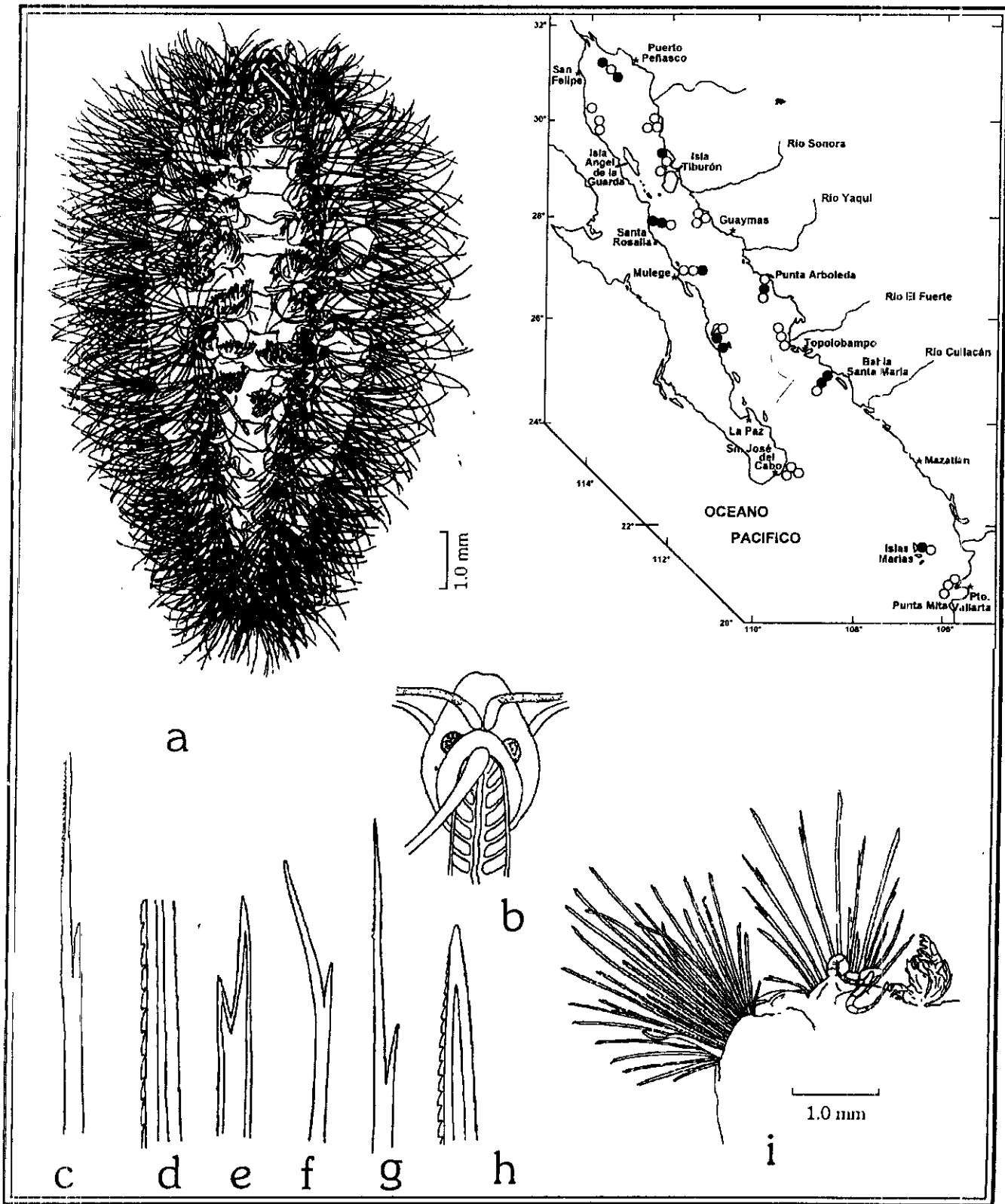
Figura 15.1. Chloeia entypa : a) Organismo completo, vista dorsal; b) Región anterior, vista dorsal; c) Seta notopodial dorsal aserrada; d) Porción media de la seta notopodial; e) Región distal de una seta; f) Seta notopodial lisa del parapodio 4; g) seta notopodial aserrada de, parapodio 10; h) Punta de una seta notopodial del parapodio medio; i) Parapodio del setígero 8. Figs. b-h: tomadas de Hartman 1940.
