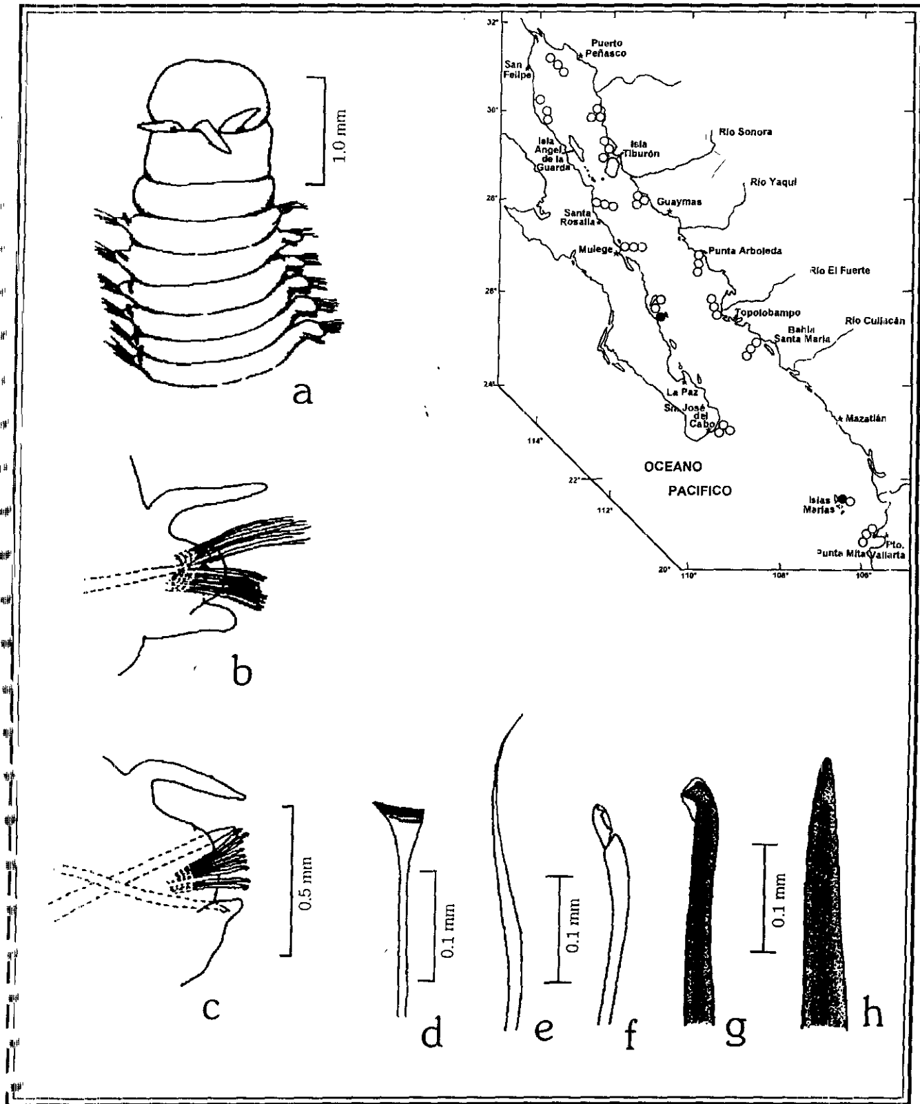
Figura 18.4. Lysidice ninetta : a) Región anterior, vista dorsal; b) Parapodio anterior; c) Parapodio posterior; d) Seta pectinada; e) Seta limbada; f) Falcígero compuesto; g) Gancho cubierto subacicular; h) Acicula. Figs. Tomadas de Gathof 1984.
