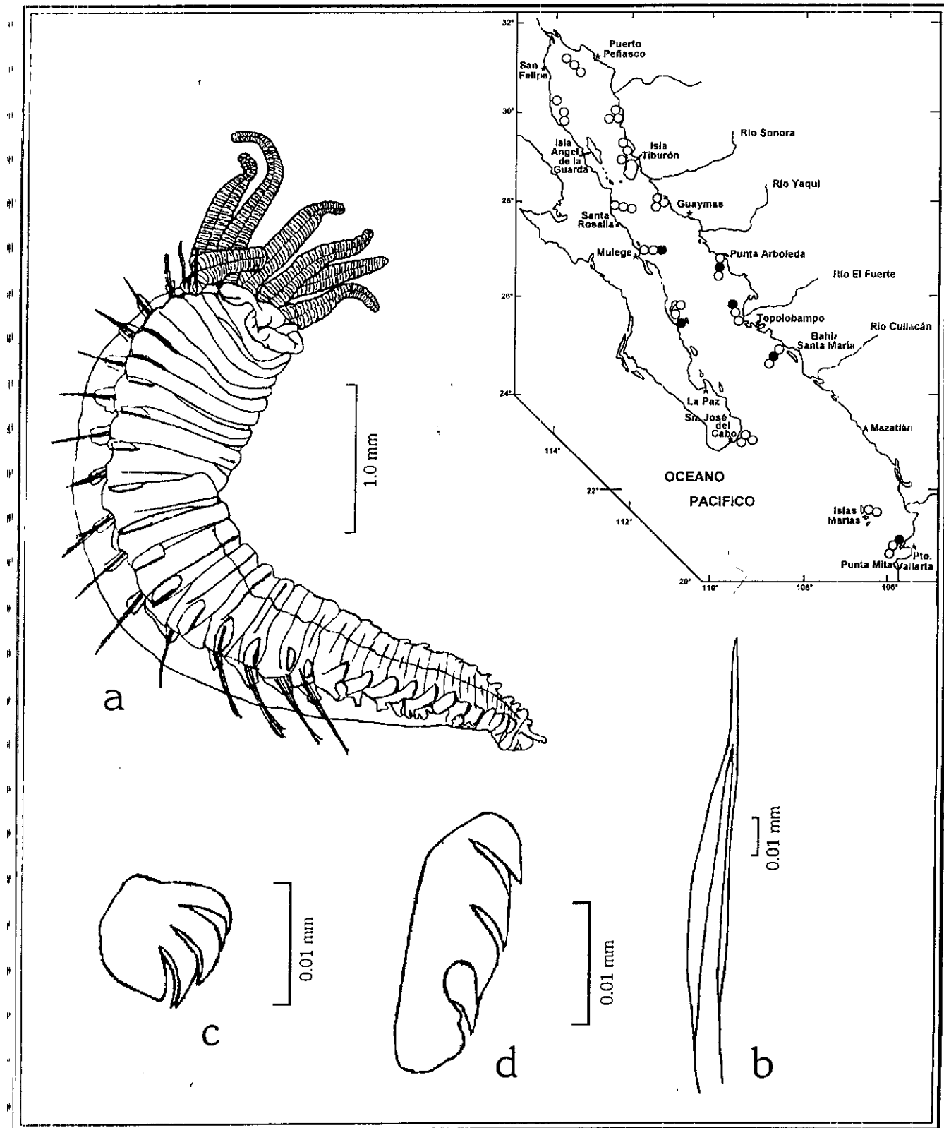
Figura 37.2. Asabellides lineata : a) Región anterior, vista lateral; b) Seta abdominal. c) Gancho abdominal; d) Gancho torácico.
