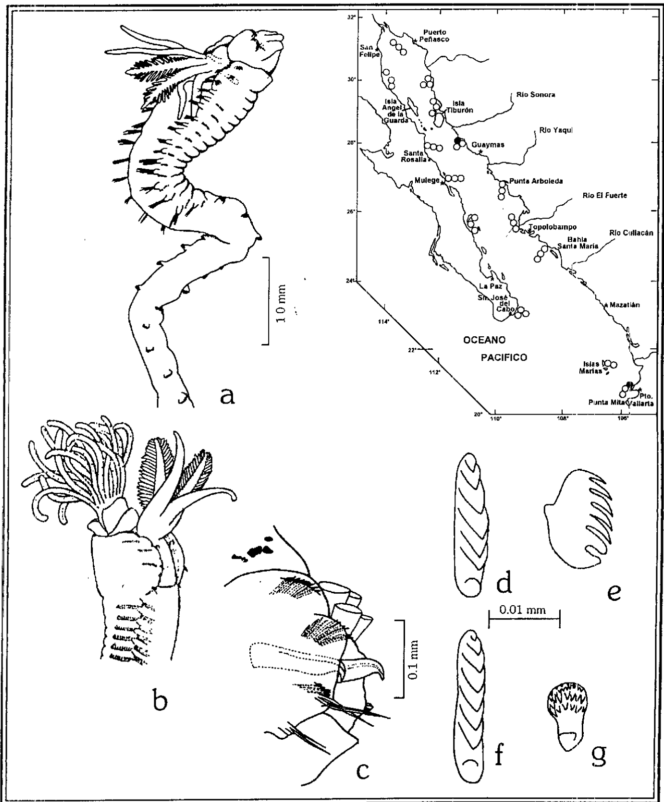
Figura 37.4. Isolda pulchella : a) Región anterior, vista dorsolateral; b) Región anterior, con tentáculos; c) Segmentos III y VI, vista lateral; d, e) Uncino torácico; f) Uncino abdominal anterior; g) Uncino abdominal posterior. Figs. a, c-g: tomadas de Uebelacker 1984; Fig. b: tomada de Day 1967.
