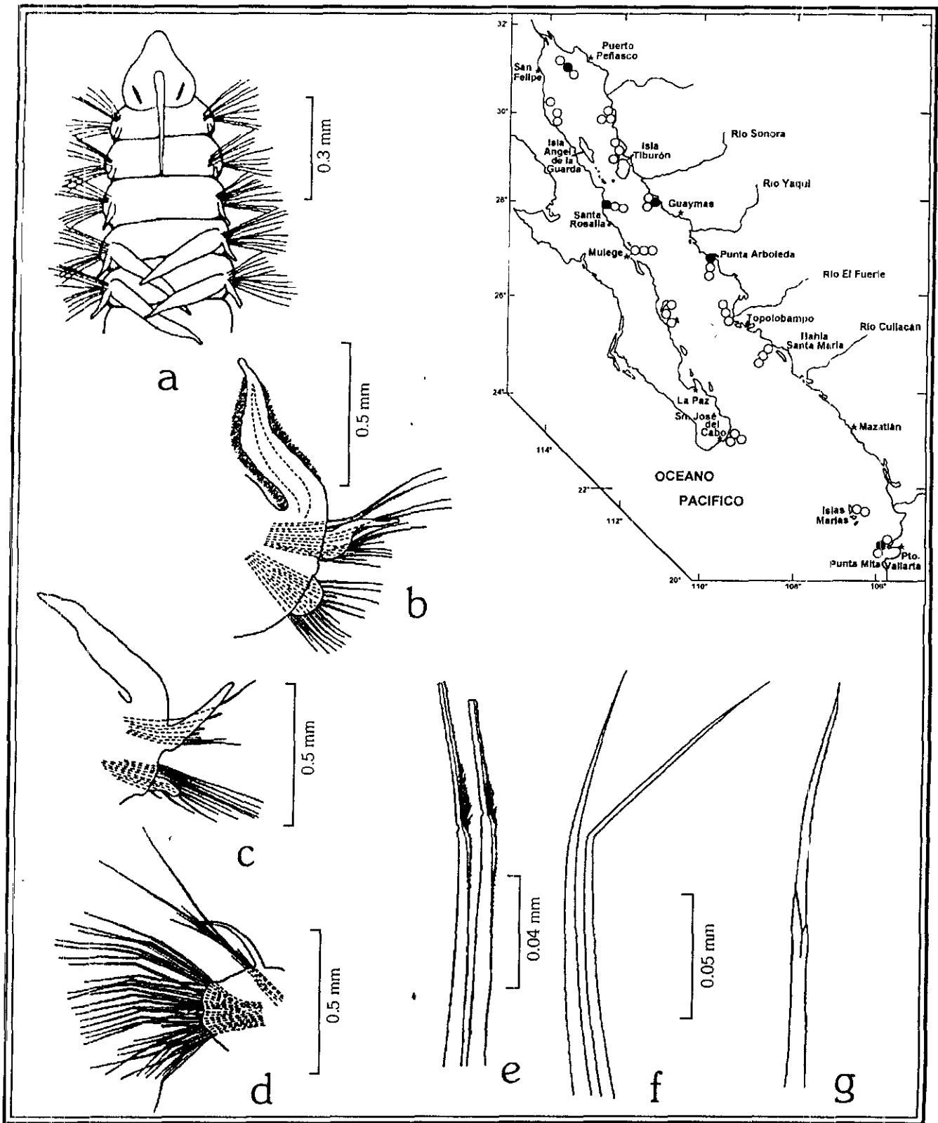
Figura 23.7. Aricidea (Aricidea) fragilis : a) Región anterior, vista dorsal; b) Parapodio del segmento 12; c) Parapodio del segmento 17; d) Parapodio posterior; e) Neurosetas pseudoarticuladas postbranquiales; f) Setas modificadas; g) Neurosetas posterior, mostrando la articulación. Figs. a, e: tomadas de Gaston 1984; Figs. b-d, f: tomadas de Strelzov 1979; Fig. g: tomada de Hartman 1947.
