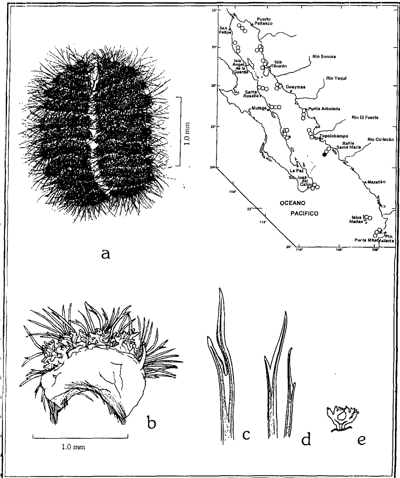
Figura 16.1. Euphrosine arctia : a) Organismo completo, vista dorsal; b) Parapodio 10; c) Notoseta bifida; d) Neuroseta simple bífida; e) Branquia típica. Figs. c-e: tomadas de Johnson 1897.
