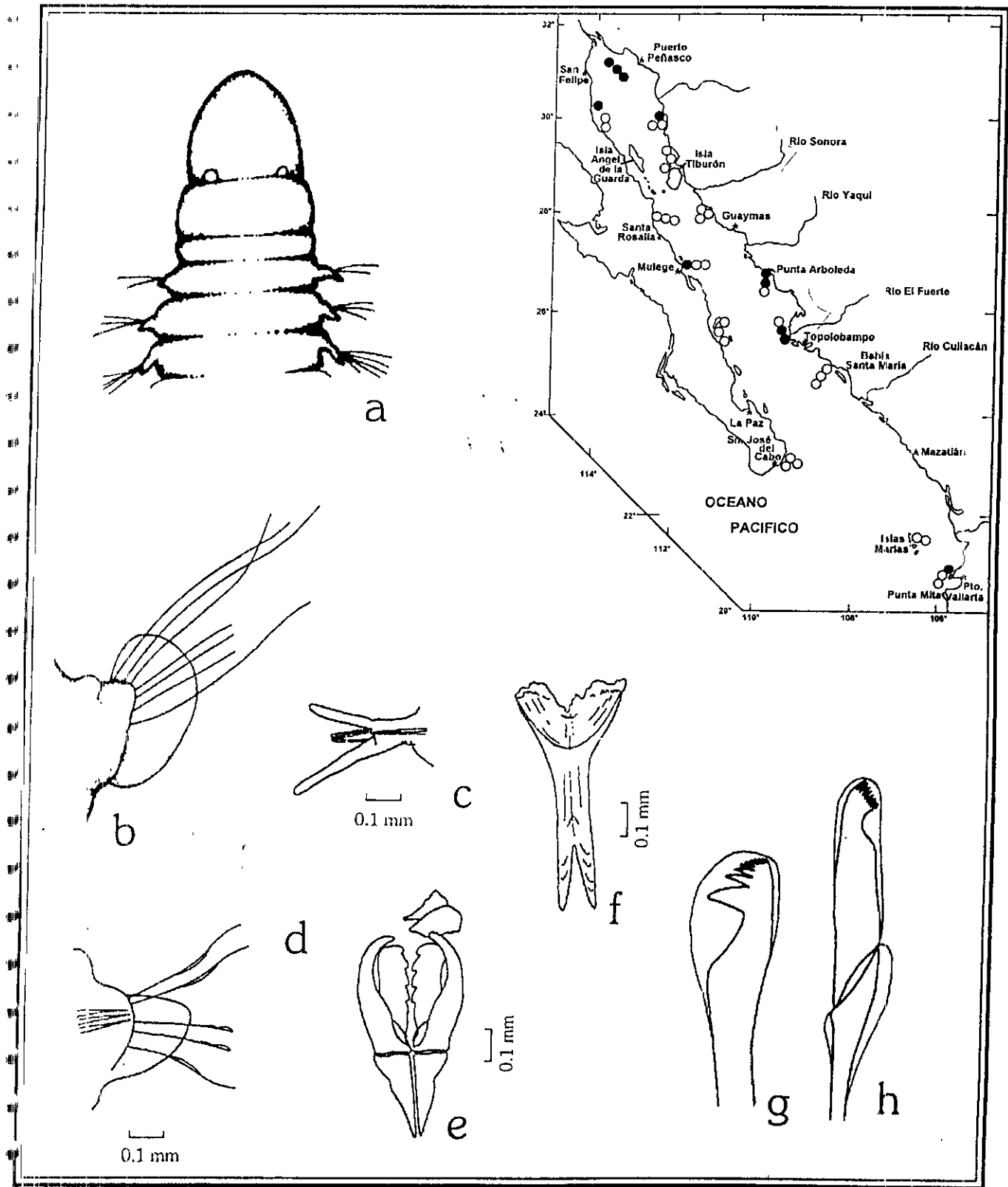
Figura 19.6. Lumbrineris cruzensis : a) Región anterior, vista dorsal; b) Parapodio 5; c) Parapodio posterior con lóbulos pre- y postsetales largos; d) Parapodio anterior; e) Maxila; f) Mandíbulas; g) Gancho cubierto simple, setífero 70; h) Gancho cubierto compuesto, setífero 5. Figs. a, b, g, i) tomadas de Fauchald 1970; Figs. c, e, f: tomadas de Hartman 1944d
