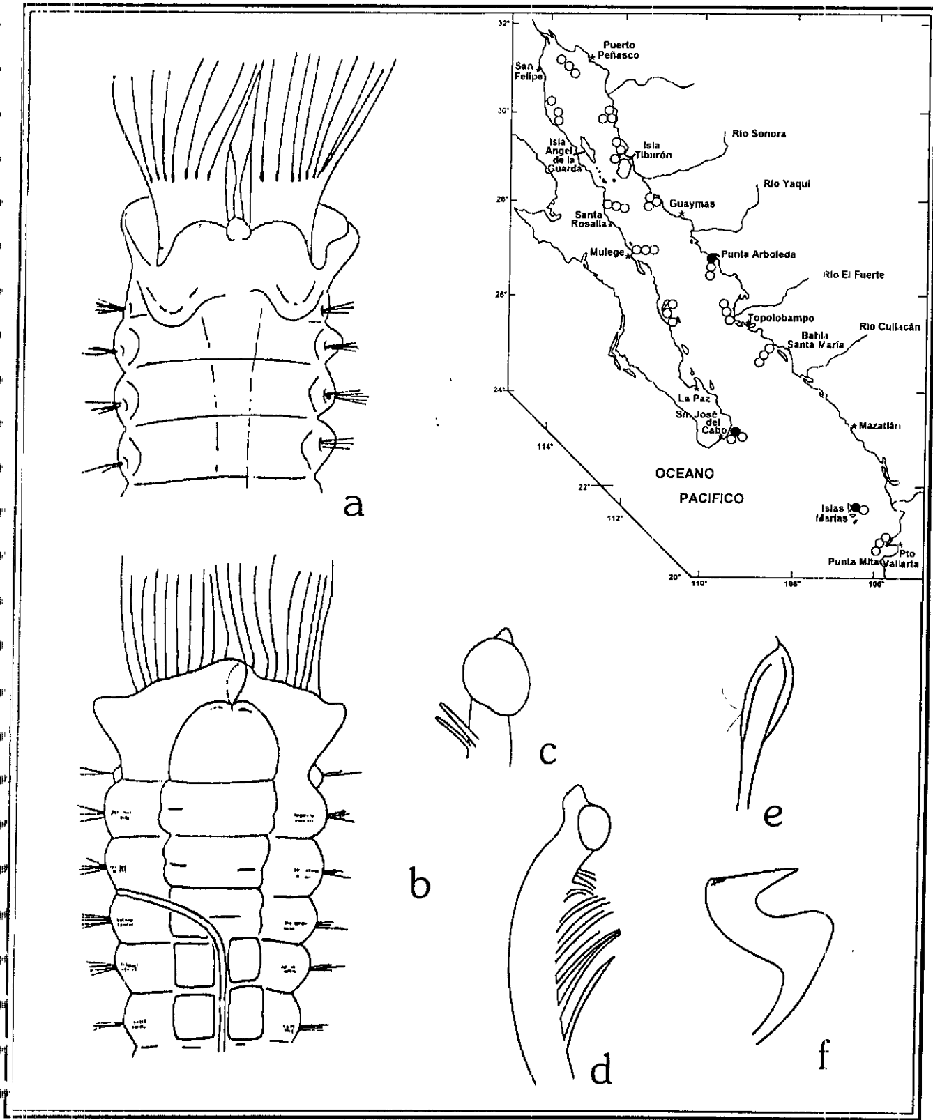
Figura 40.3. Megalomma circumspectum : a) Región anterior con base tentacular y collar de membrana; b) Collar membranoso y cojinetes anteriores; c) Ojos compuestos; d) Los mismos ojos vistos por otro lado; e) Seta espatulosa torácica; f) Cresta de uncino torácico. Figs. a-d: tomadas e Harman 1969; Figs. e, f: tomadas de Moore 1923.
