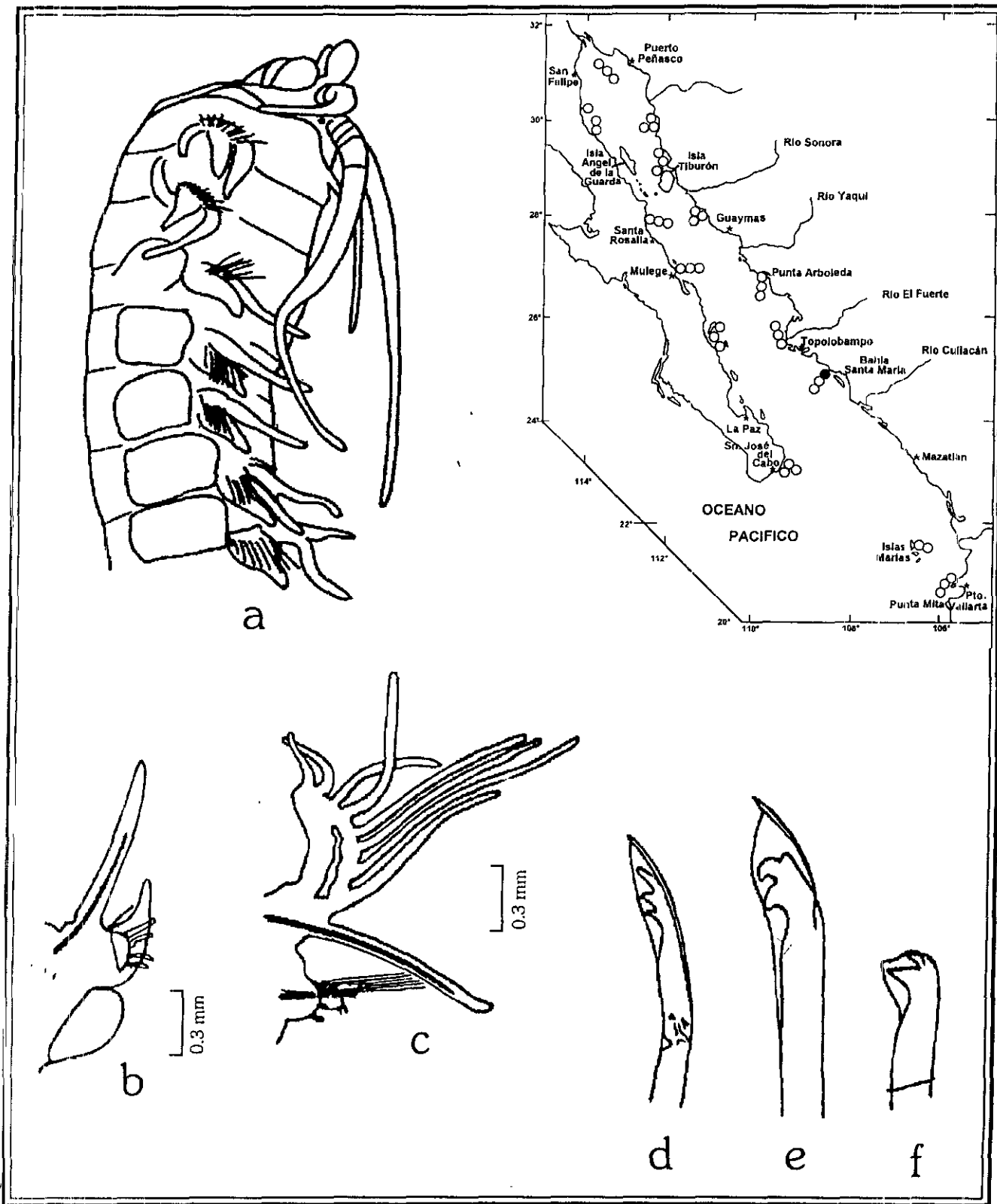
Figura 17.9. Kinbergonuphis microcephala : a) Región anterior, vista lateral; b) Segmento 2; c) Segmento 58 con branquias; d) Gancho cubierto trífido; e) Gancho subacicular; f) Gancho subacicular trífido. Fig. a: tomada de Fauchald 1982; Figs. b-f: tomadas de Hartman 1944.
