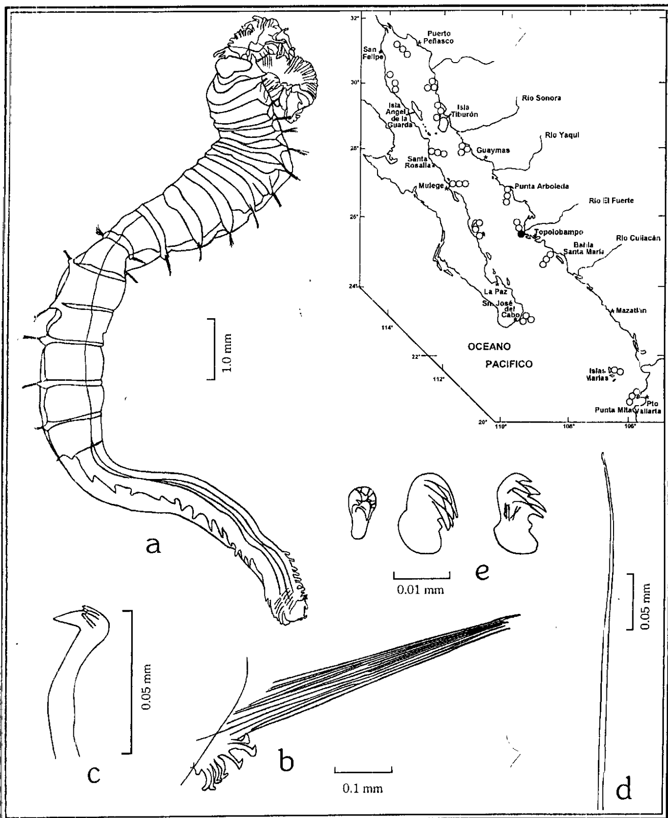
Figura 38.2. Terebellides reishi : a) Organismo completo, vista lateral; b) Setígero 6; c) Gancho del setígero 6, vista lateral; d) Seta capilar; e) Ganchos de setígero abdominal, diferentes vistas.
