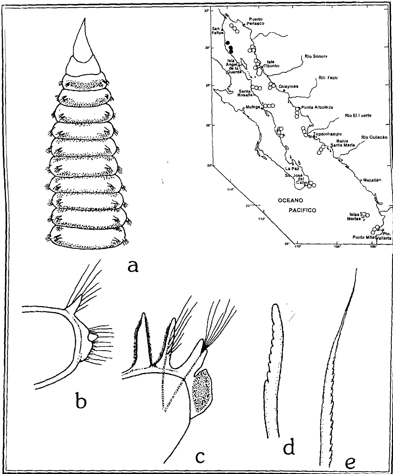
Figura 22.9. Scoloplos (Scoloplos) texana : a) Región anterior, vista dorsolateral; b) Décimo setífero torácico; c) Parapodio posterior; d) Gancho neuropodial torácico; e) Notoseta furcada abdominal. Figs. a-c: tomadas de Maciolek y Holland 1978; Figs. d, e: tomadas de Taylor 1984.
