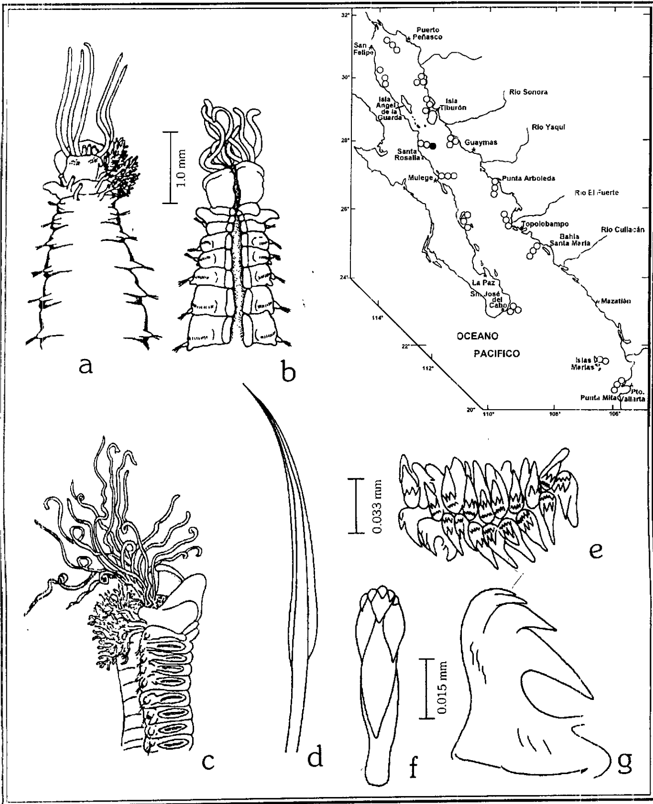
Figura 39.3. Lanice conchilega : a) Región anterior, vista dorsal; b) Región anterior, vista ventral; c) Región anterior, vista lateral; d) Notoseta; e) Uncino torácico posterior, con doble arreglo de líneas; f) Uncino torácico del setífero 2, vista frontal; g) El anterior, vista lateral. Figs. a, b, d-g: tomadas de Kritzler 1984; Fig. c: tomada de Fauvel 1927 y Mc. Intosh 1922.
