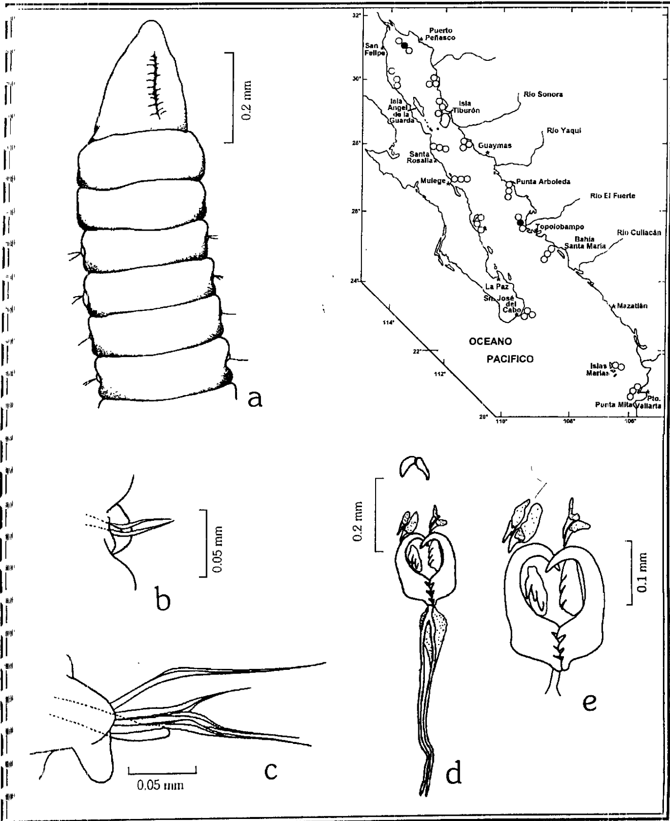
Figura 20.3. Drilonereis longa : a) Región anterior; b) Parapodio del setígero 6; c) Parapodio de región media del cuerpo; d) Aparato maxilar; e) Detalle de la maxila. Figs. Tomadas de Uebelacker 1984.
