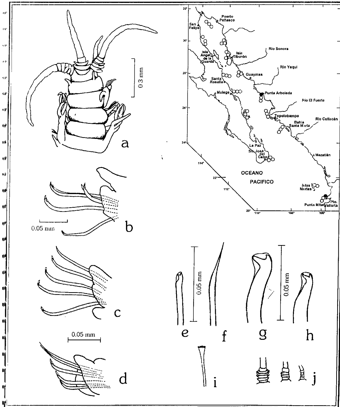
Figura 17.3. Diopatra papillata : a) Región anterior, vista dorsal; b) Parapodio del primer setígero; c) Setígero 2; d) Setígero 3; e) Gancho bidentado del setígero 6; f) Seta limbada del setígero 6; g) Gancho subaciclar superior; h) Gancho subaciclar inferior; i) Seta pectinada; j) Ceratóforos de los tetáculos occipitales. Figs. a-h: tomadas de Gathof 1984; Figs. i-j: tomadas de Fauchald 1968.
