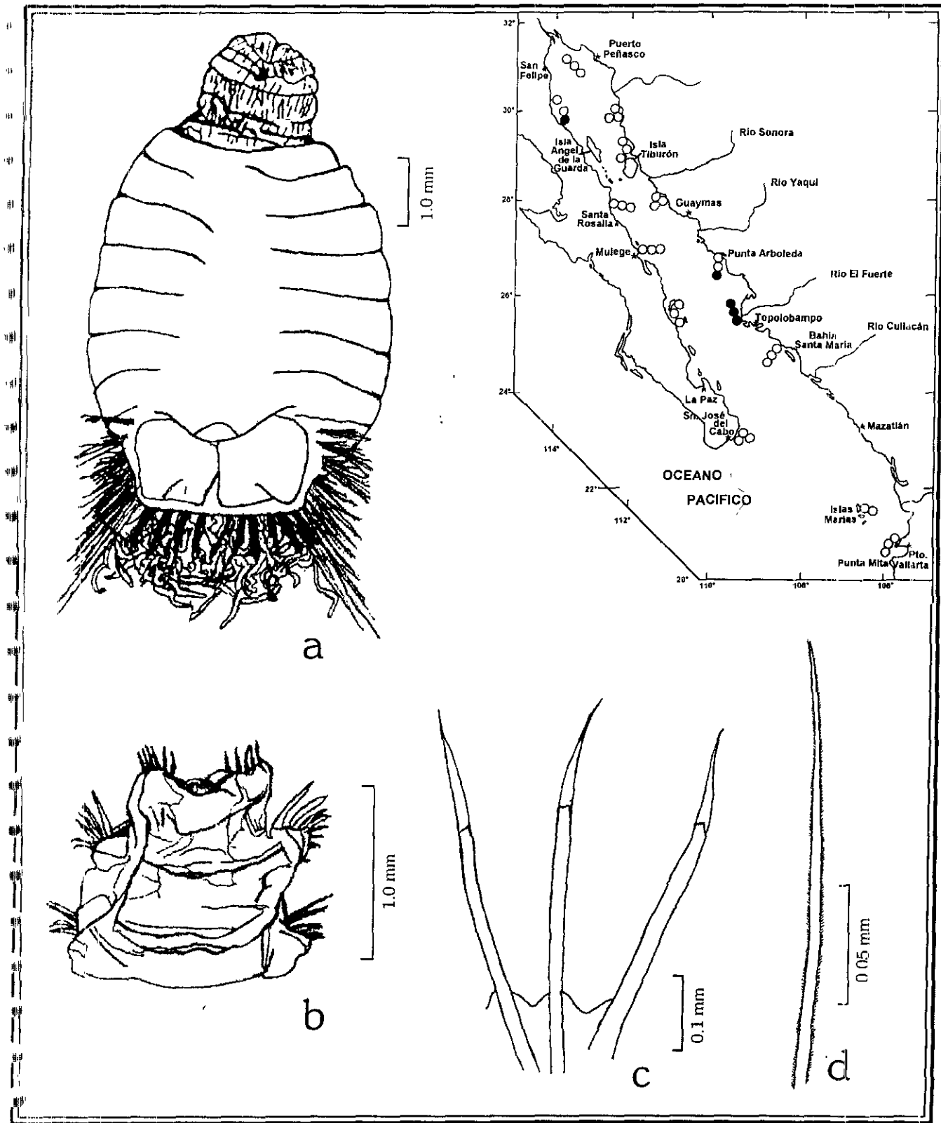
Figura 33.1. Sternaspis fossor : a) Organismo completo, vista ventral; b) Porción anterior; c) Espinas gruesas de setígeros anteriores; d) Setas puntiguas posteriores.
