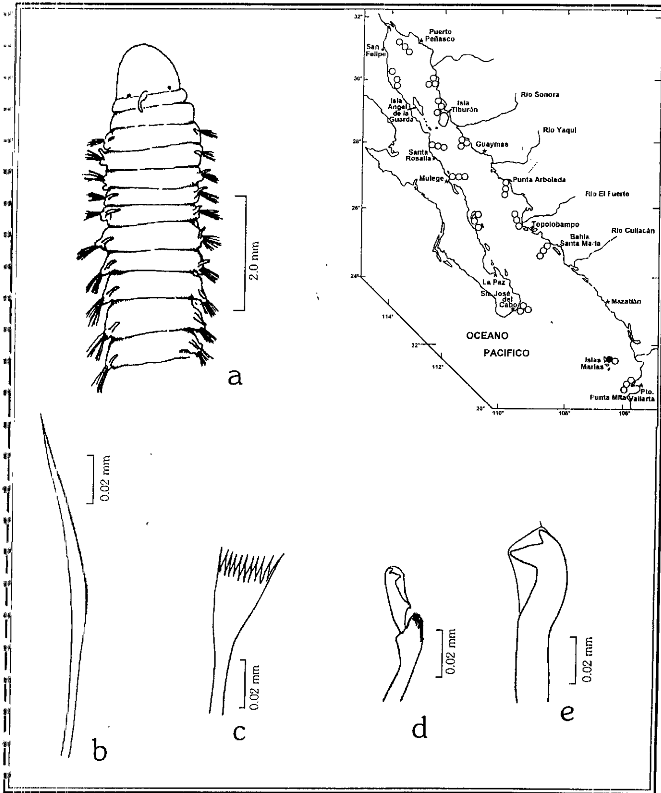
Figura 18.7. Nematonereis hebes : a) Región anterior, vista dorsal; b) Seta limbada; c) seta pectinada; d) Falcígero compuesto; e) Gancho cubierto subacicular. Figs. Tomadas de Gathof 1984.
