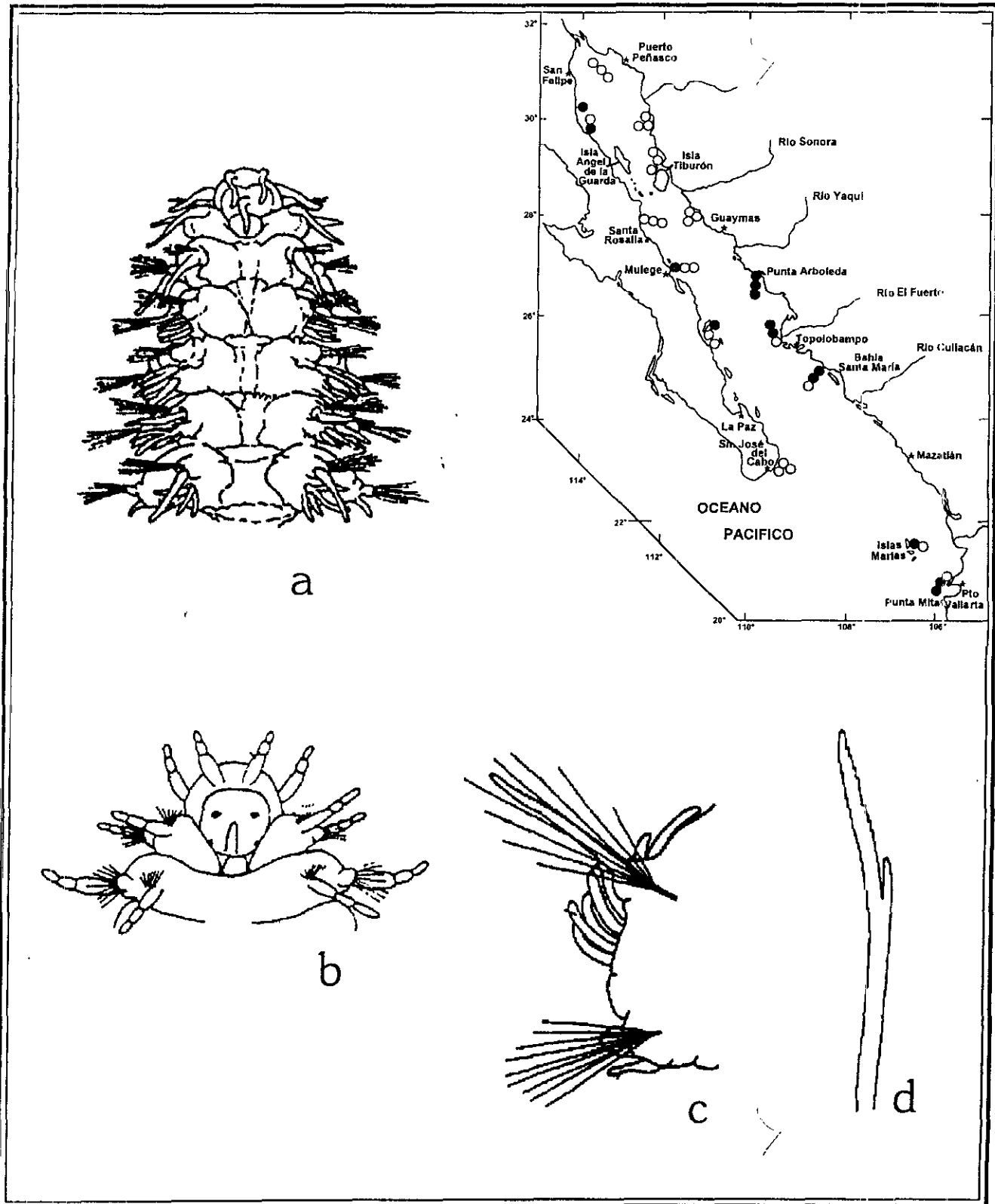
Figura 15.3. Linopherus ambigua : a) Región anterior, vista ventral; b) Región anterior., vista dorsal; c) Región anterior, vista anterior; d) Neuroseta furcada. Fig. a: tomada de Hartman 1968, Figs. b-d: tomadas de Gardiner 1976.
