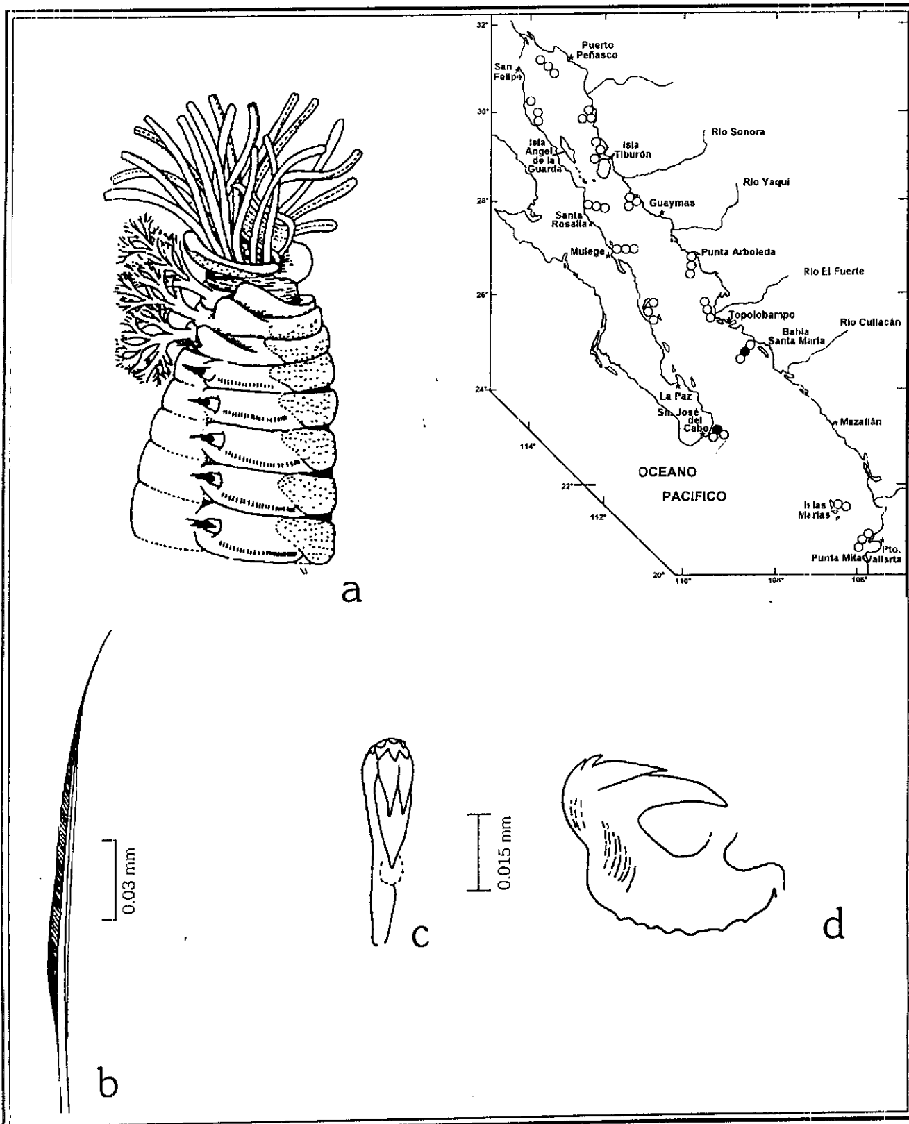
Figura 39.2. Eupolytmnia nebulosa : a) Región anterior, vista lateral; b) Notoseta; c) Uncino torácico, vista frontal; d) Uncino torácico, vista lateral: Fig. a: tomada de Day 1967; Figs. b-d: tomadas de Kritzler 1984.
