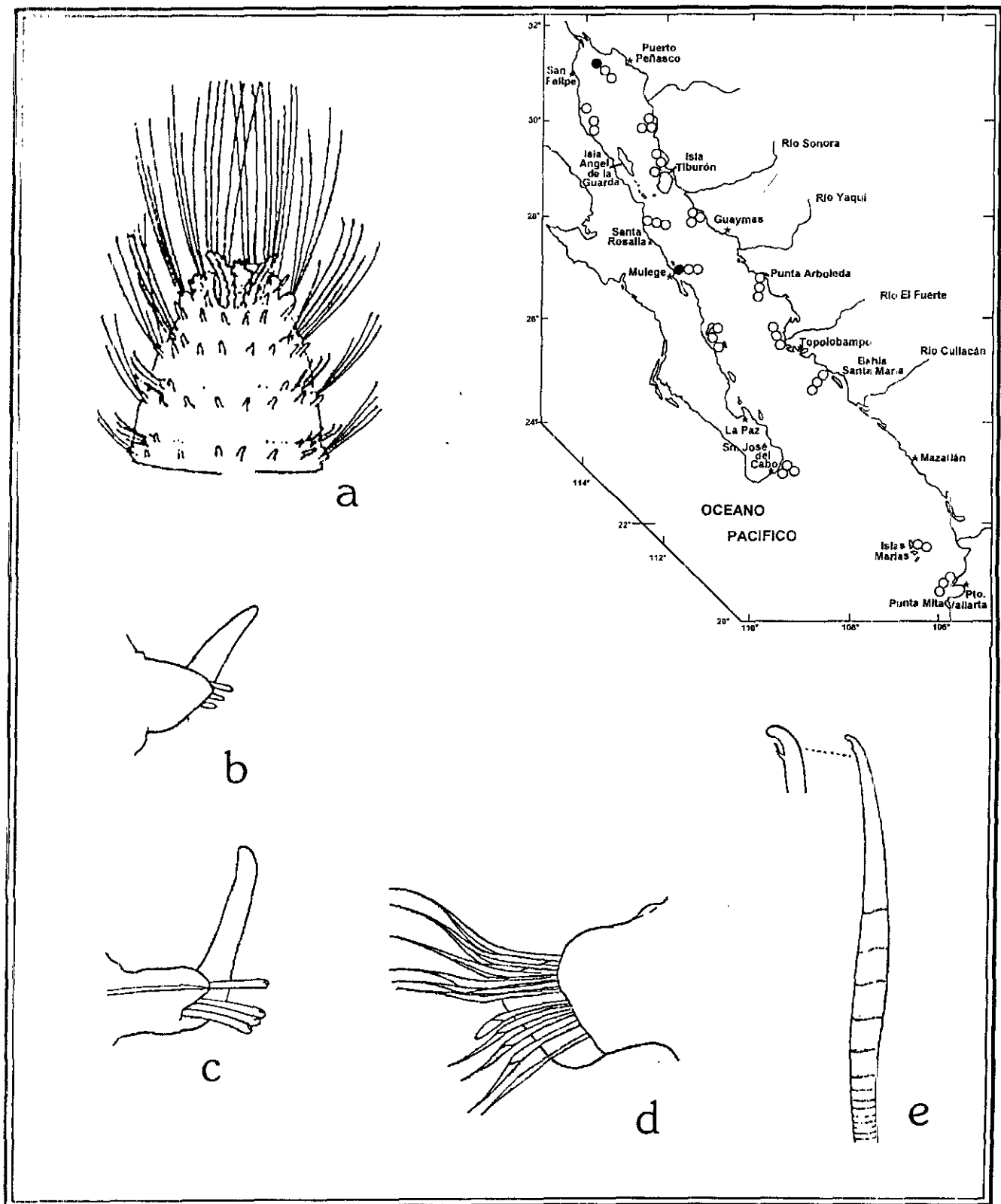
Figura 31.3. Piromis arenosus : a) Organismos completo; b) Región anterior, vista ventral; c) Región distal de una seta de un segmento medio; d) Parapodio de la región media; c) Neuropodio; f) Ganchos neuropodiales. Figs. a, b, f: tomadas de Day 1967; Figs. c e: tomadas de Hartman 1948a.
