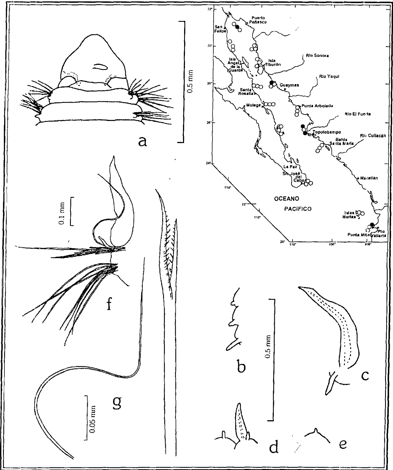
Figura 23.9. Cirrophorus furcatus . a) Región anterior, vista dorsal; b) Lóbulos parapodiales de los tres primeros segmentos; c-e) Lóbulos notopodiales y branquias de los segmentos medios; f) Seta furcada notopodial, abdominal; g) Setígero veinte; b) Seta capilar delgada. Figs. a-e: tomadas de Strelzov 1979; Fig. f: tomada de Hartman 1969.
