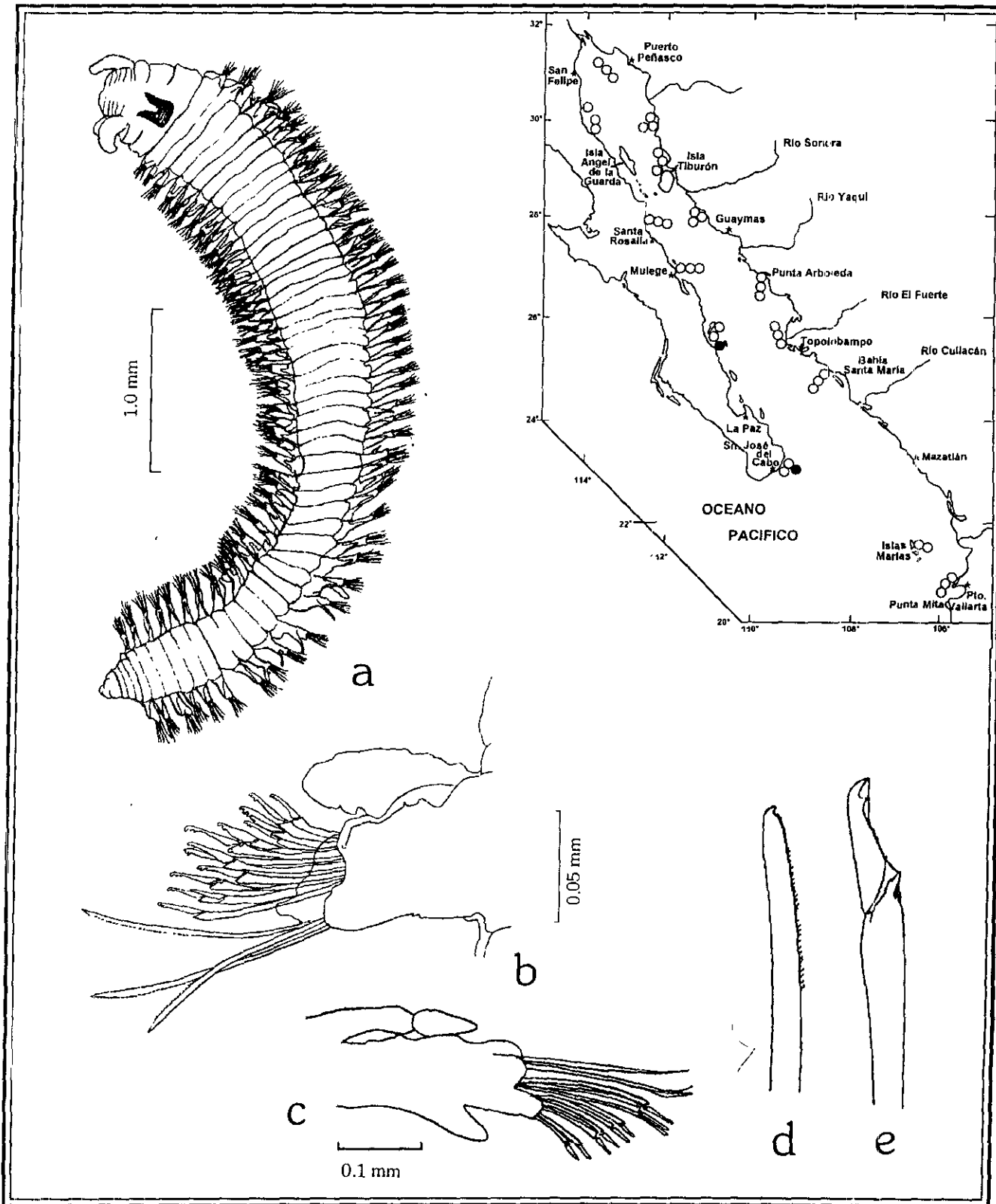
Figura 21.1. Dorvillea moniloceras : a) Organismos completo, vista dorsal; b) Primer parapodio; c) Parapodio medio; d) Falcígero con terminación bífida; e) Seta subacicular compuesta. Figs. d, e: tomadas de Moore 1909.
