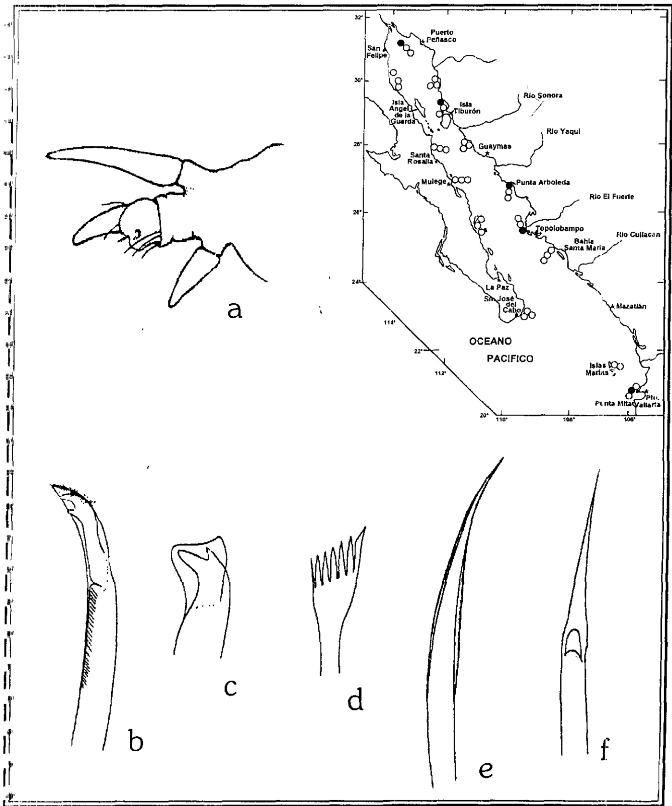
Figura 17.4. Diopatra splendidissima : a) Primer parapodio; b) Gancho bifido cubierto; c) Gancho subacicular; d) Seta pectinada; e) Seta limbada aserrada lateralmente; f) Acicula. Fig. a: tomada de Fauchald 1968; Figs. b-f: tomadas de Moore 1904.
