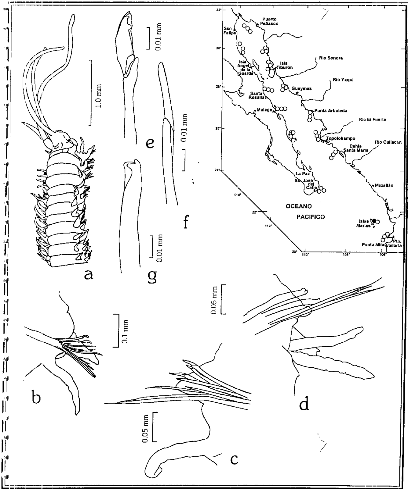
Figura 17.15. Mooreonuphis ca. guadalupensis : a) Región anterior, vista dorsal; b) Setígero 4; c) Setígero 11; d) Setígero 20; e) Gancho pseudocompuesto del setígero 4, vista lateral; f) Espiniger compuesto, setígero 11; g) Gaucho subacicular, setígero 20.
