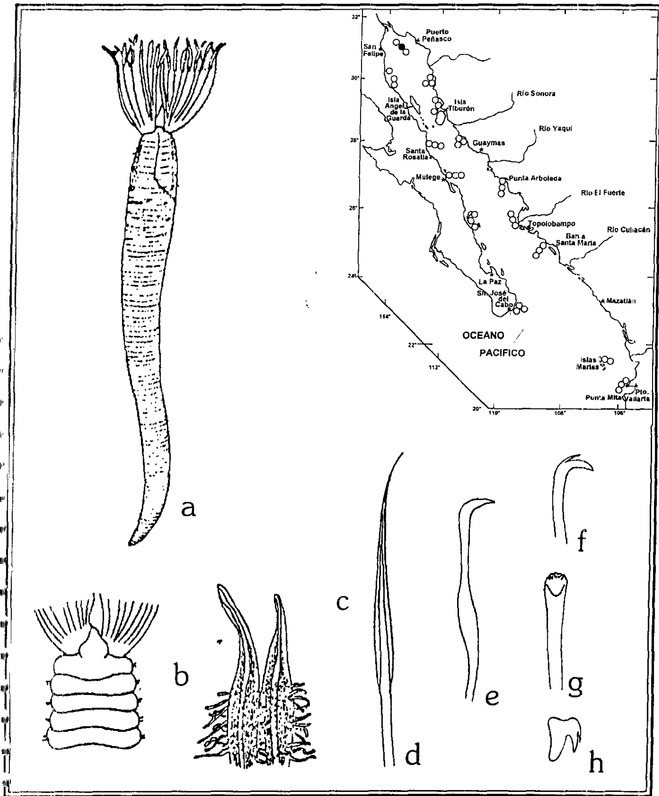
Figura 40.5. Myxicola infundibulum : a) Organismo completo, vista ventral; b) Región anterior con radiolos cortados, vista ventral; c) Región distal de los radiolos con pínulas; d) Seta capilar; Uncino torácico; f) Uncino torácico con punta bífida; g) Uncino torácico, vista frontal; Uncino abdominal, vista lateral. Figs. a-c, e, f, h: tomadas de Fauvel 1927; Figs. d, g: tomadas de Day 1967.
