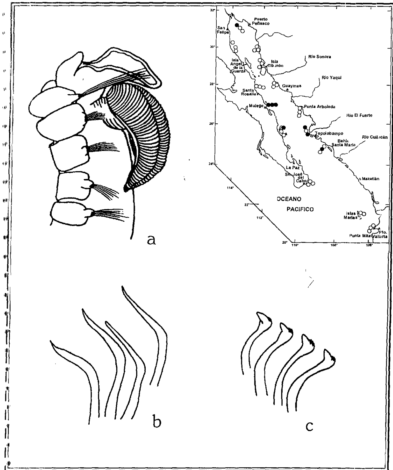
Figura 38.1. Terebellides californica : a) Región anterior, vista lateral; b) Seta acicular, setígero 6; c) Uncino torácico. Figs. Tomadas de Williams 1984.
