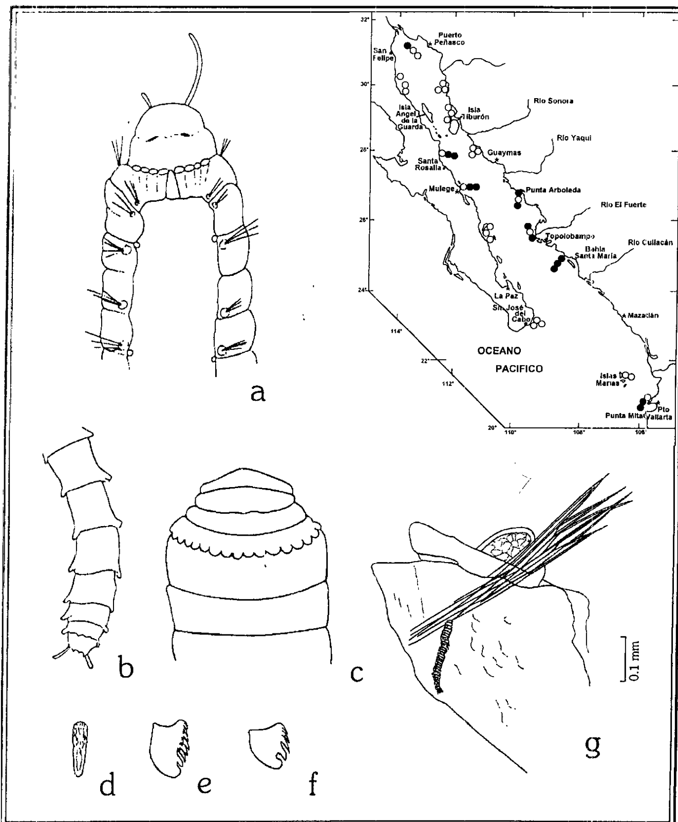
Figura 37.5. Lysippe annectens : a) Región anterior con branquias, vista dorsal; b) Región posterior con cirro anal, vista ventral; c) Región anterior, vista ventral; d) Uncino torácico, vista frontal; e) Uncino torácico vista lateral; f) Uncino abdominal, vista lateral; g) Setígero 9, torácico. Fig a-f: tomadas de Moore 1923.
