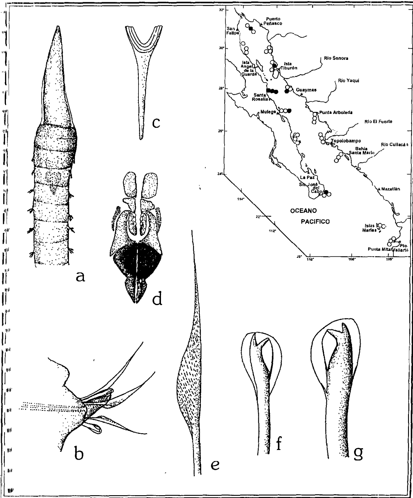
Figura 19.3. Lumbrinerides acutiformis : a) Región anterior, vista dorsal; b) Parapodio medio; c) Mandíbula; d) Aparato maxilar; e) Seta limbada; f) Gancho cubierto bidentado de un setígero anterior g) Gancho cubierto bidentado de un setígero posterior. Figs. Tomadas de Gallardo 1968.
