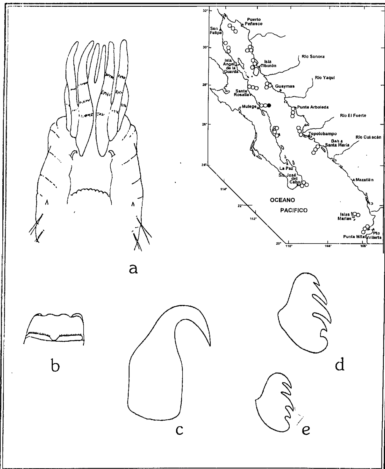
Figura 37.6. Melinna oculata : a) Región anterior, con branquias; b) Prostomio; c) Espina nual; d) Uncino torácico; e) Uncino abdominal. Figs. Tomadas de Hartman 1969.
