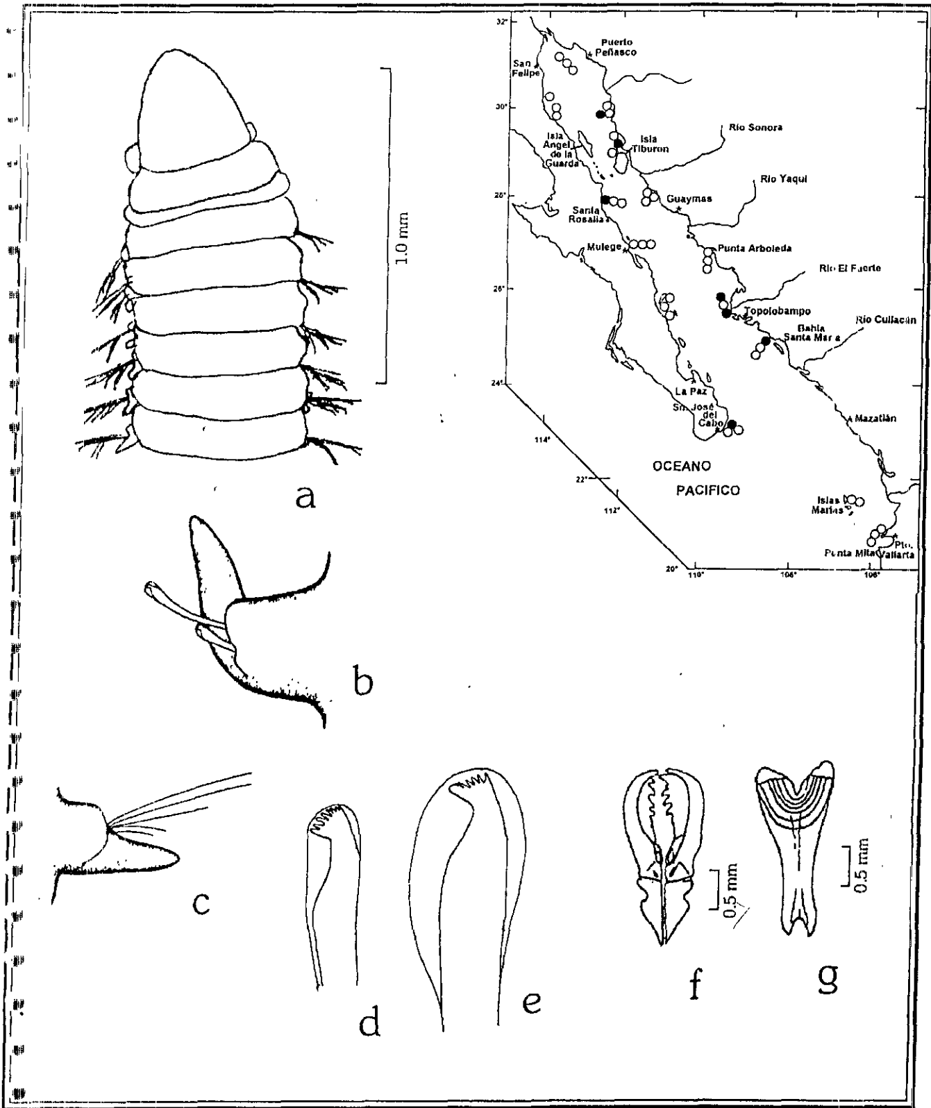
Figura 19.11. Lumbrineris tetraura : a) Región anterior, vista dorsal; b) Parapodio 5; c) Parapodio posterior, d) Gancho cubierto simple, setífero 5; e) Gancho cubierto simple, setífero posterior f) Maxila; g) Mandíbula. Figs. b-e: tomadas de Fauchald 1970; Figs. f, g: tomadas de Hartman 1944d.
