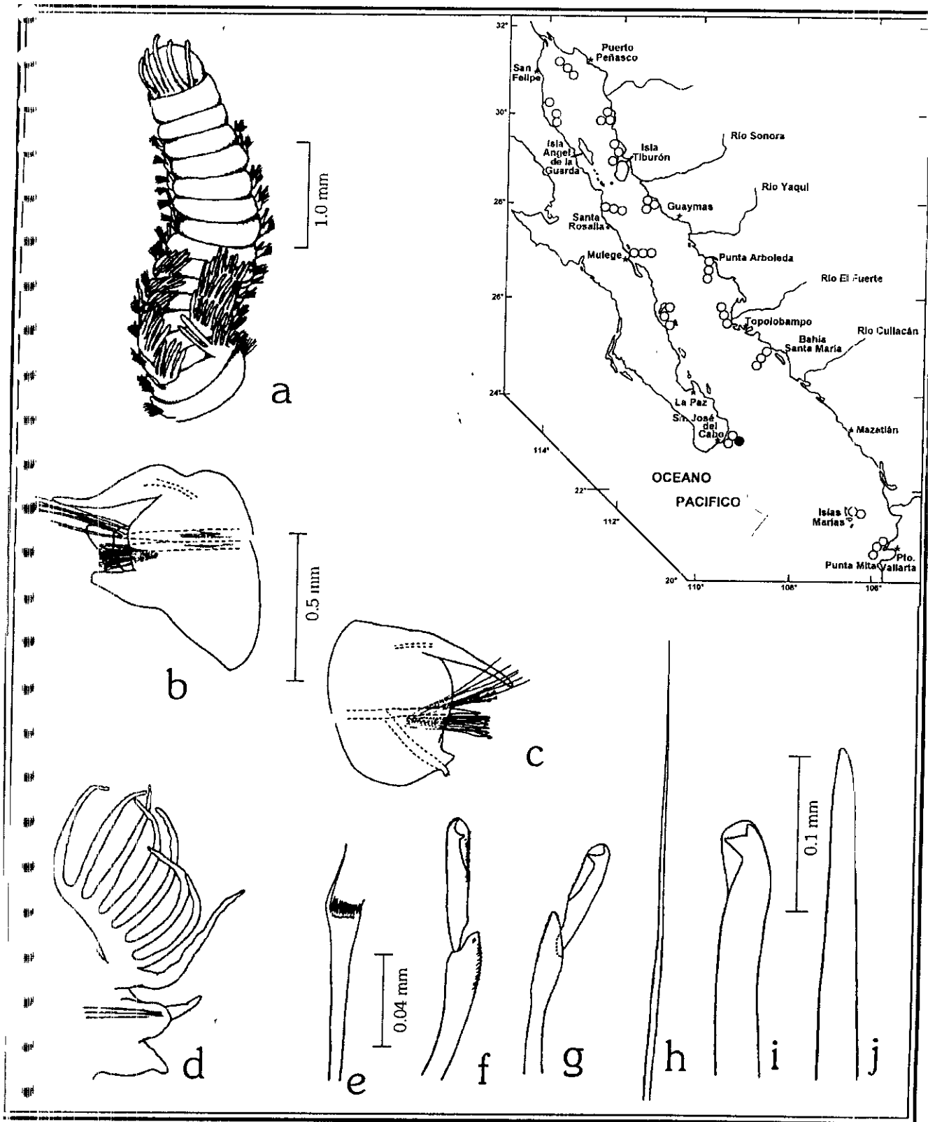
Figura 18.5. Marphysa conferta : a) Región anterior, vista dorsal; b) Parapodio anterior; Parapodio posterior; d) Parapodio con branquias; e) Seta pectinada; f) Falcígero compuesto anterior; g) Falcígero compuesto posterior; h) Seta capilar; i) Gancho cubierto subacicular; Acicula. Figs. a-g, e-j: tomadas de Gathof 1984; Fig. d: tomada de Moore 1911.
