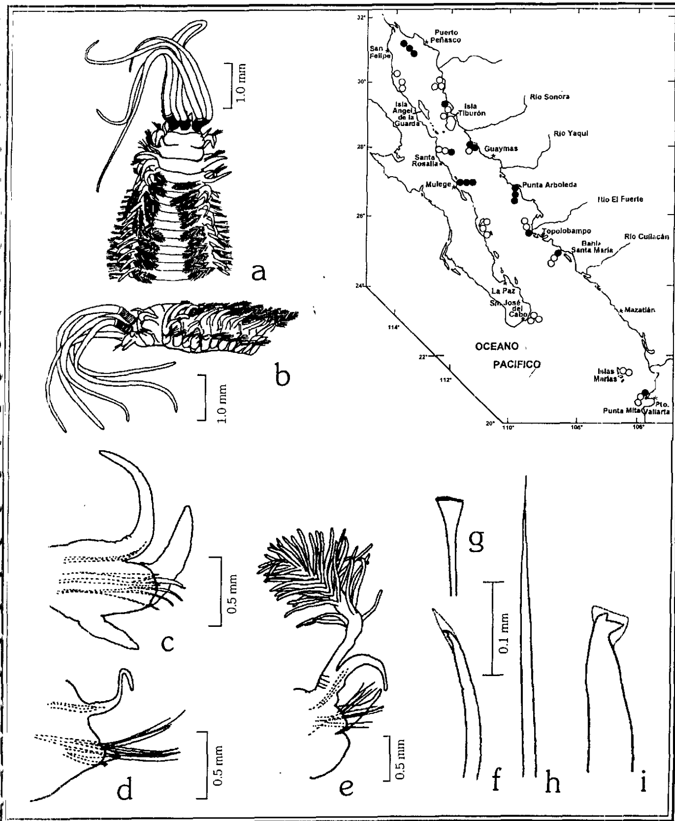
Figura 17.5. Diopatra tridentata : a) Región anterior, vista dorsal; b) Región anterior, vista lateral; c) Setígero 2; d) Setígero 25; e) Setígero 5; f) Gancho pseudocompuesto del setígero 2; g) Seta pectinada; h) Seta capilar; i) Gancho subacicular. Figs. Tomadas de Gathof 1984.
