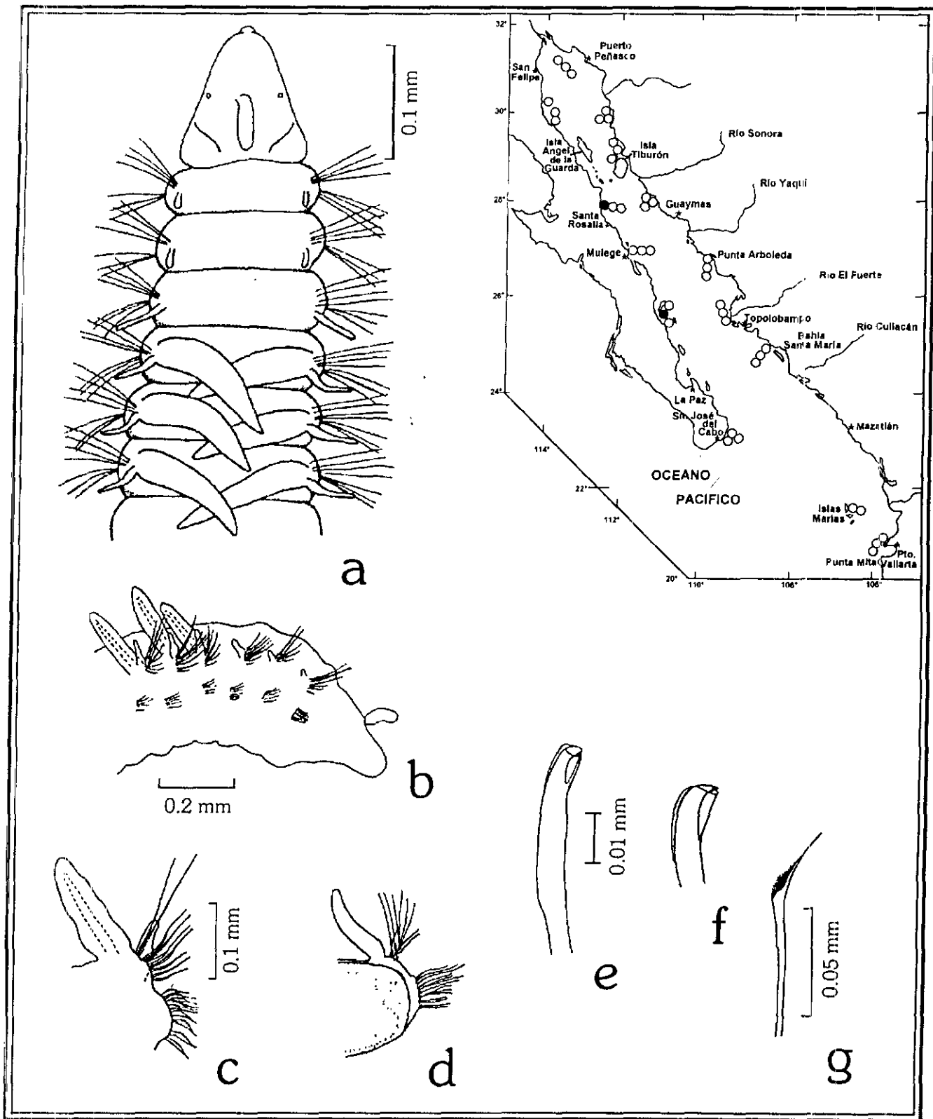
Figura 23.2. Aricidea (Acmira) cerrutti : a) Región anterior, vista dorsal; b) Región anterior, vista lateral; c) Parapodio del segmento 7; d) Parapodio branquial; e, f) Setas modificadas; g) Neuroseta del segmento 8. Fig. a: tomada de Gaston 1984; Figs. b, c, e-g: tomadas de Strelzov 1979; Fig. d: tomadas de Day 1967.
