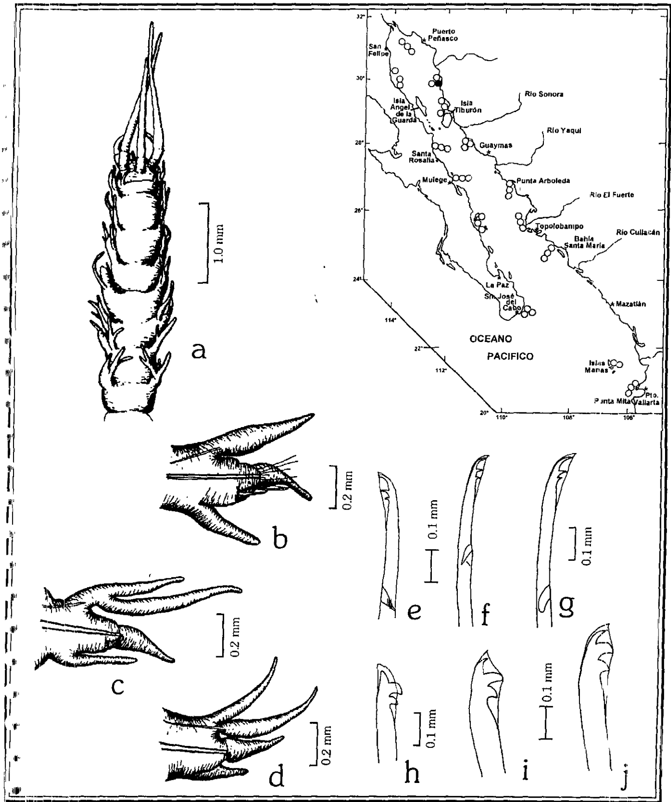
Figura 17.1.3. Kinbergonuphis virgata : a) Región anterior, vista dorsal; b) Setígero 3; c) Setígero 9; d) Setígero 12; e) Gancho pseudocompuesto del setígero 3; f, g) Ganchos pseudo compuesto del setígero 7; h-j) Ganchos largos, (h) Del setígero 12; (i) Del setígero 6; (j) Del setígero 7. Figs. Tomadas de Fauchald 1980.
