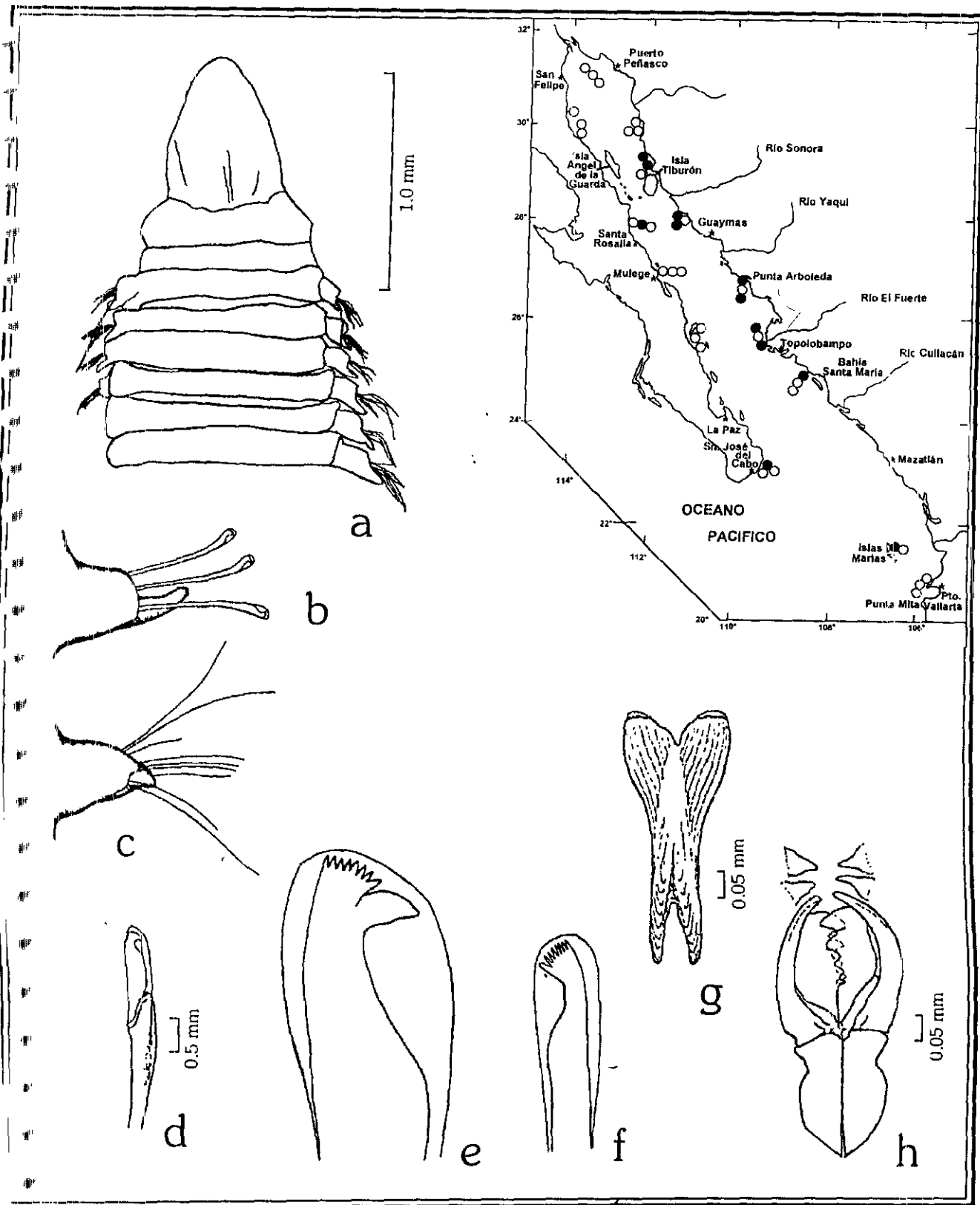
Figura 19.9. Lumbrineris limicola : a) Región anterior, vista dorsal; b) Parapodio posterior; c) Parapodio 5; d) Gancho cubierto compuesto; e) Gancho cubierto simple, setífero posterior; f) Apendice de un gancho compuesto, setífero 5; g) Mandíbula; h) Maxila. Figs. d, g, h: tornadas Hartman 1944d; b, c, e, f: tomadas de Fauchald 1970.
