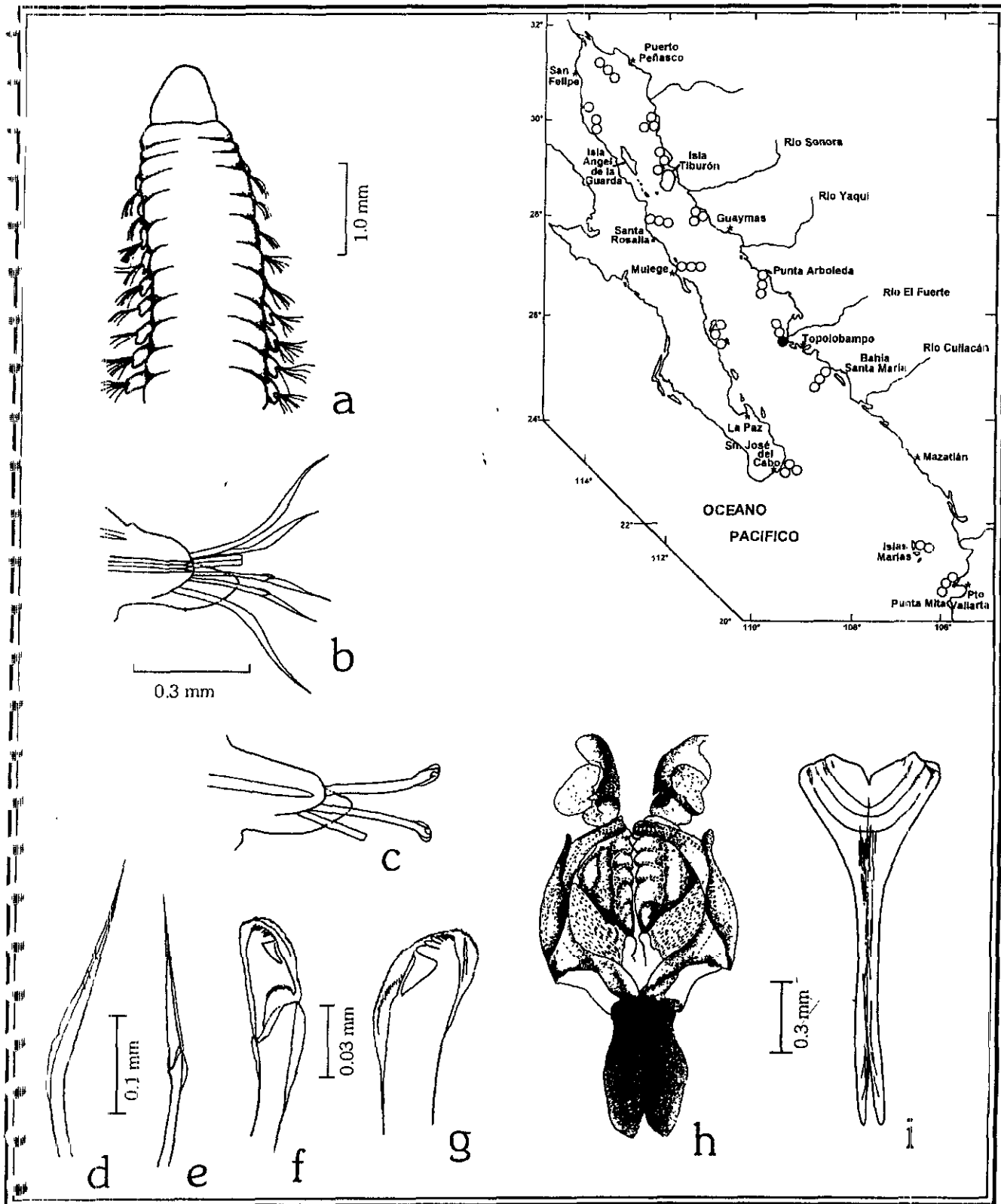
Figura 19.2. Lumbricalus dayi : a) Región anterior, vista dorsal; b) Parapodio del setígero 10; c) Parapodio de la región media; d) Seta limbada simple de] setígero 6; e) Seta limbada compuesta del setígero 6; f) Gancho cubierto compuesto de la región media; g) Gancho cubieto simple de la región posterior; h) Maxila; i) Mandíbula. Figs. Tomadas de Uebelacker 1984.
