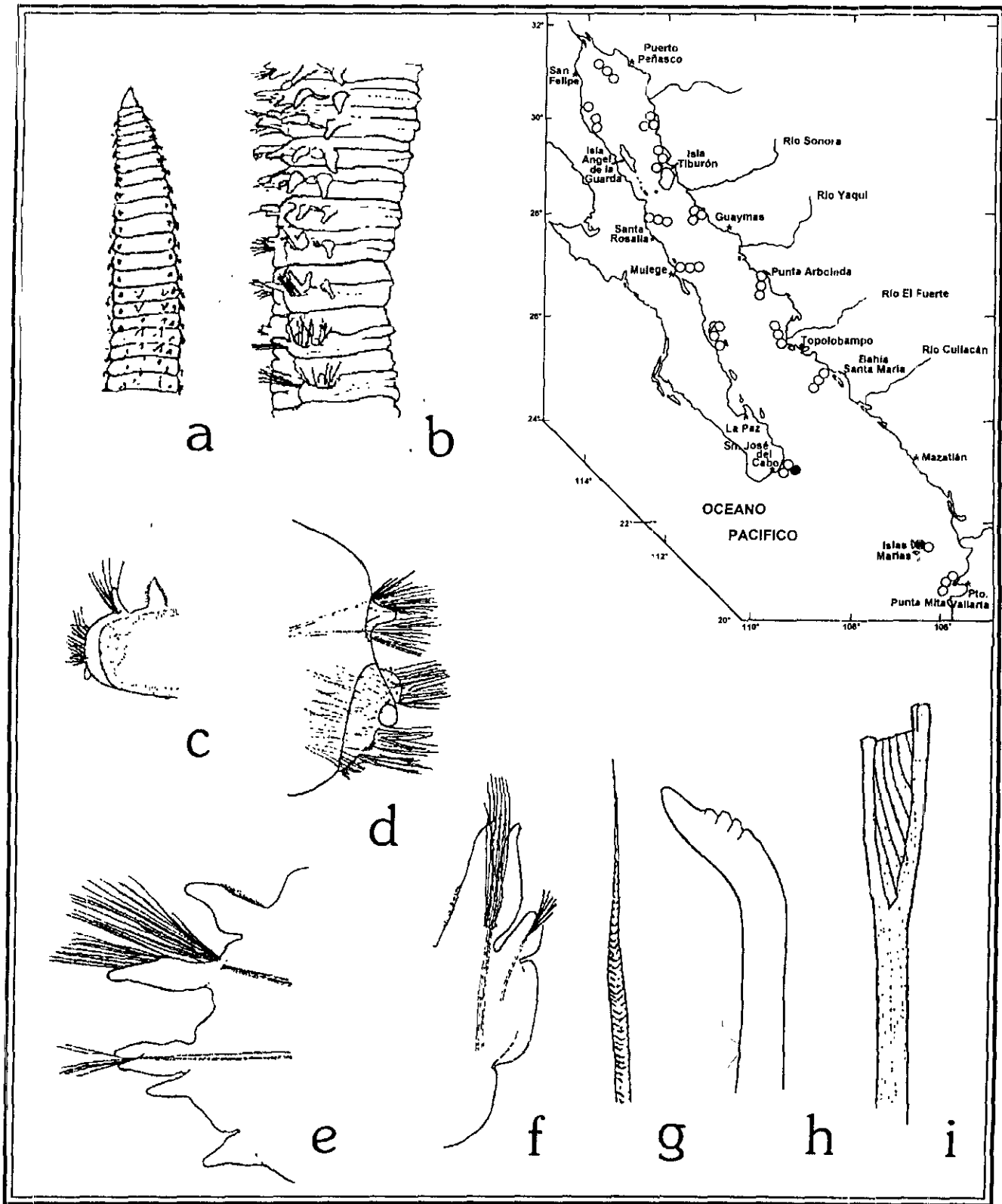
Figura 22.7. Scololoplos (Scoloplos) armiger : a) Región anterior, vista dorsal; b) Región de transición, segmentos 16 a 24; c) Parapodio torácico; d) Doceavo parapodio torácico; e) Parapodio abdominal anterior; f) Parapodio abdominal medio; g) Seta crenulada; h) Gancho neuropodial torácico. i) Seta furcada abdominal. Figs. a, g: tomadas de Fauvel 1927; Figs. c, i: tomadas de Day 1967; Figs. b, d, e, f, h: tomadas de Hartman 1969.
