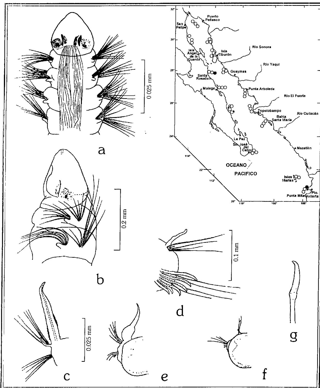
Figura 23.11. Levinsenia oculata : a) Región anterior, vista dorsal; b) Región anterior, vista dorsal; c) Parapodio del tercer segmento branquial; d) Segmento branquial; e) Parapodio anterior; f) Parapodio posterior g) Neurosetas aciculares posteriores. Figs. a-c, e: tomadas de Strelzov 1979; Figs. d, f, g: tomadas de Day 1967.
