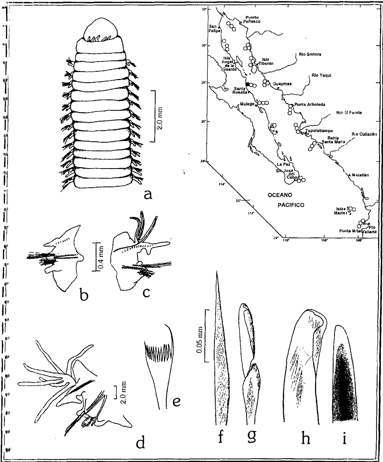
Figura 18.6. Marphysa mortenseni : a) Región anterior, vista dorsal; b) Parapodio anterior; c) Parapodio posterior; d) Parapodio con branquias; e) Seta pectinada; f) Seta limbada; g) Falcígero compuesto; h) Gancho cubierto subacicular; i) Acicula. Figs. a-c, e-i: tomadas de Gathof 1984; I d: tomada de Monro 1928b.
