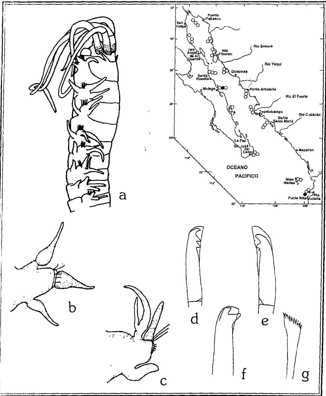
Figura 17.10. Kinbergonuphis proalopus : a) Región anterior, vista lateral; b) Primer parapodio; c) Parapodio 7; d) Gancho cubierto inferior; e) Gancho cubierto superior; f) Gancho subacicular; g) Seta pectinada, parapodio posterior. Fig. a: tomada de Fauchald 1982; Figs. b-g: tomas de Fauchald 1968
