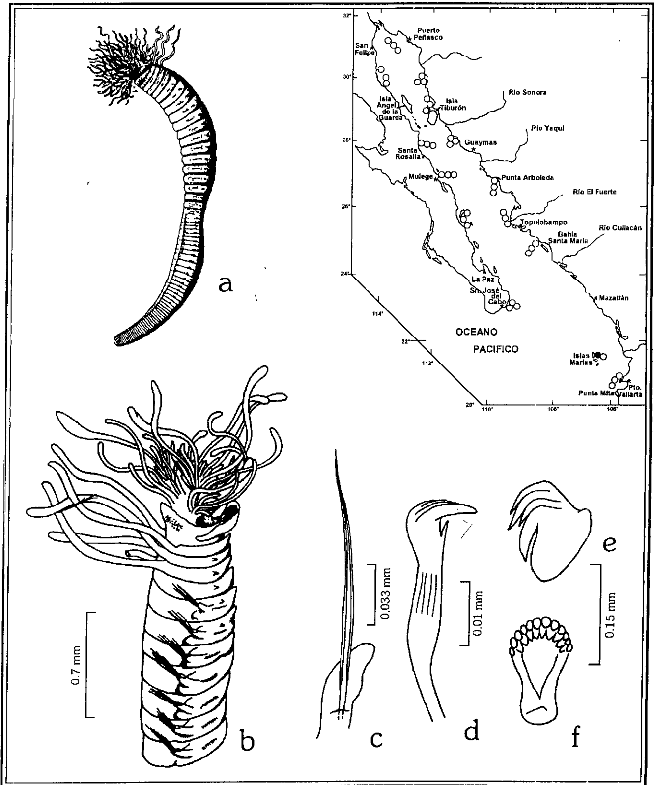
Figura 38.4. Trichobranchus glacialis : a) Organismo completo, vista lateral; b) Región anterior, vista dorsolateral; c) Notoseta proyectándose del notopodio torácico; d) Gancho rostrado neuropodial torácico; e) Uncino abdominal; f) Uncino abdominal, vista frontal. Fig. a: tomada de Holthe 1986b; b-f: tomadas de Kritzler 1984.
