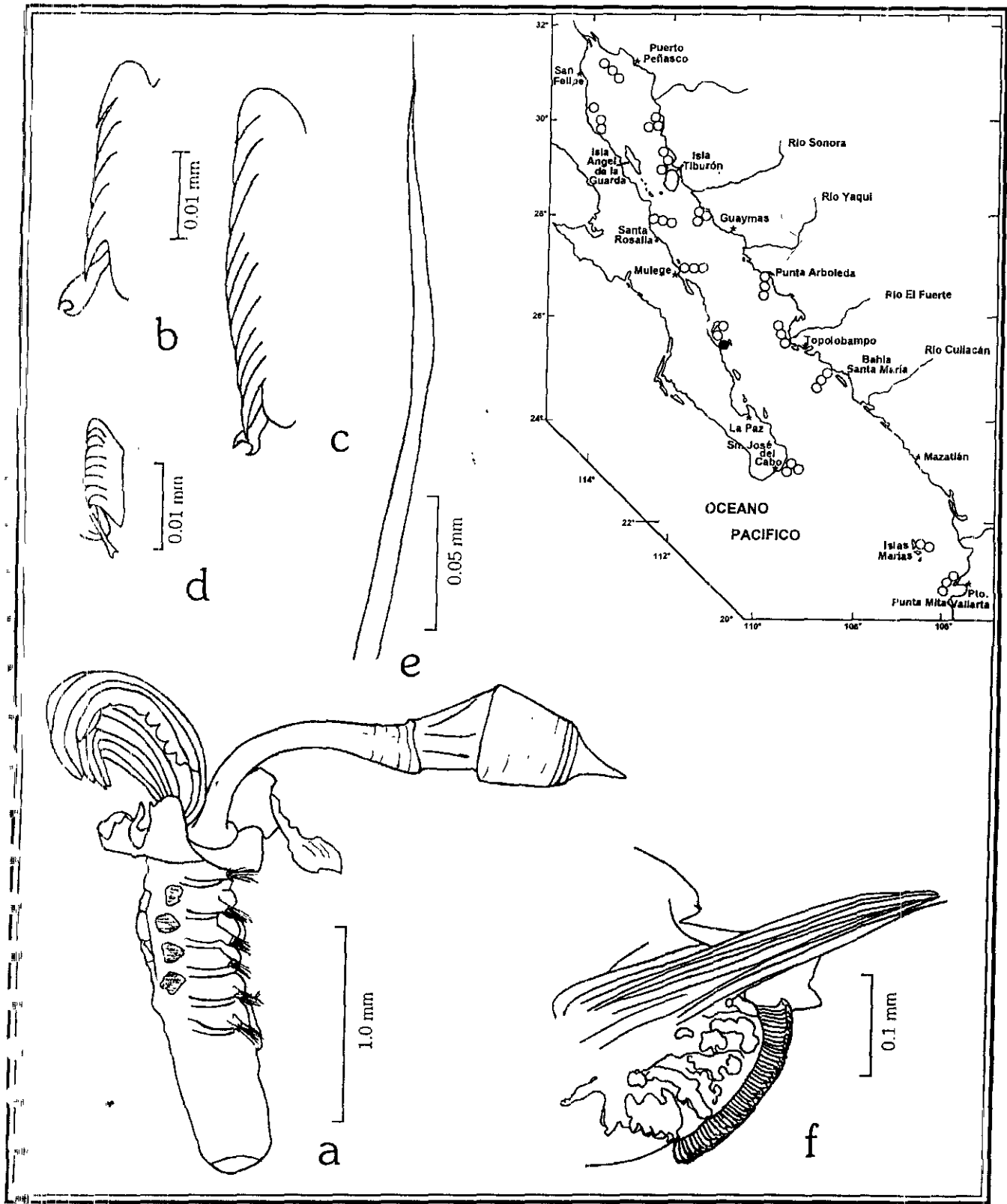
Figura 41.1. Pseudovermilia conchata : a) Organismo completo, vista lateral; b, c) Uncinos torácicos; d) Uncino abdominal; e) Seta notopodial torácica; f) Parapodio torácico.
