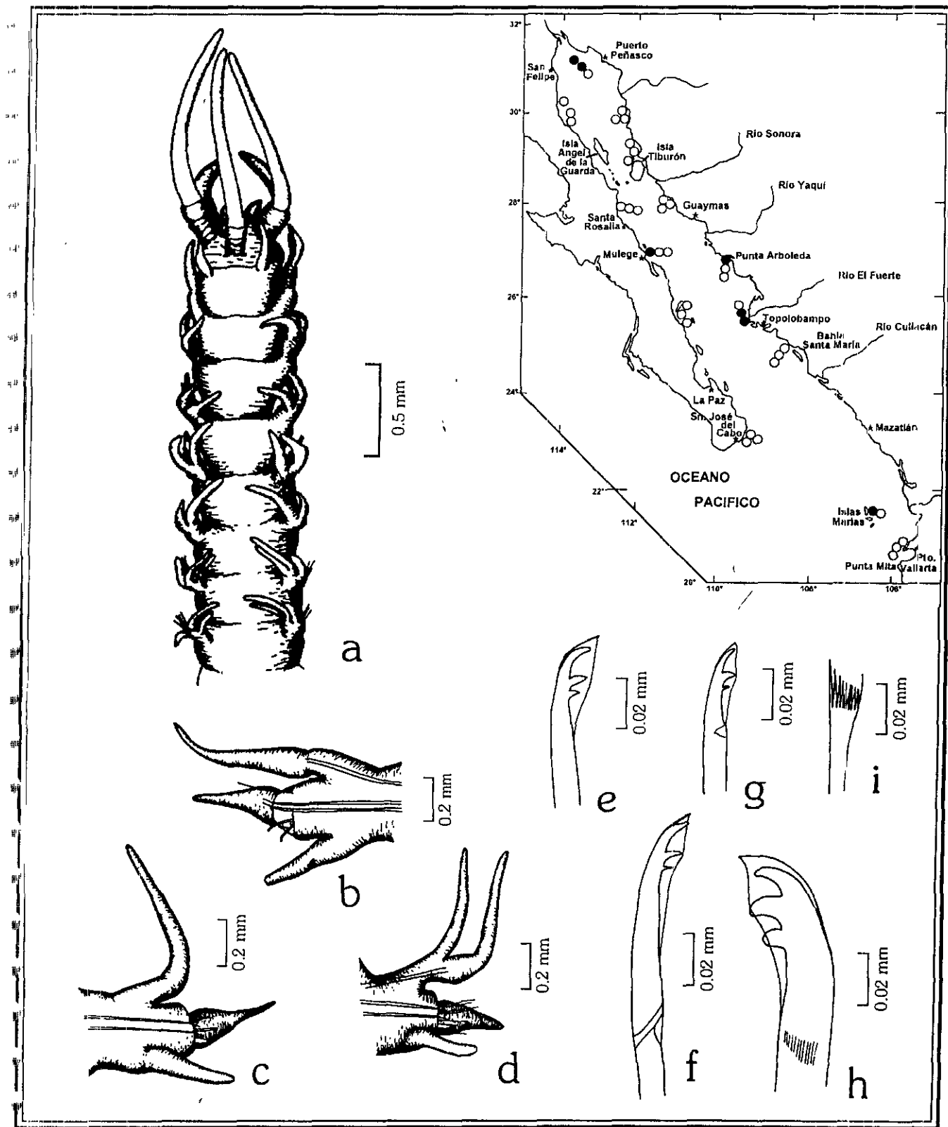
Figura 17.11. Kinbergonuphis pulchra : a) Región anterior, vista dorsal; b) Primer setígero; c) Setígero 4; d) Setígero 7; e) Gancho pseudocompuesto del setígero 4; f) Gancho i pseudocompuesto del setígero 5; g) Gancho pseudocompuesto del setígero 6; h) Gancho largo del setígero 4; i) Seta pectinada. Figs. Tomadas de Fauchald 1980.
