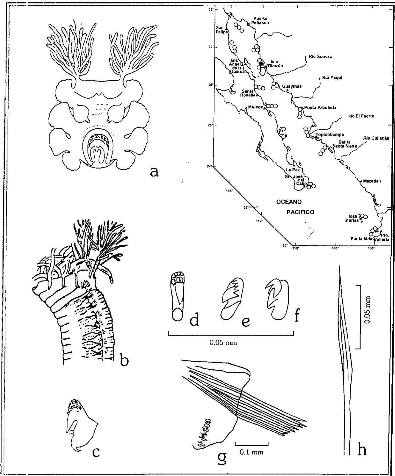
Figura 39.5. Scionella japonica : a) Región anterior, con tentáculos removidos, vista frontal; b) Región anterior, vista lateral; c) Uncino torácico, vista lateral; d) Uncinos torácicos, vista frontal lateral; e) Parapodio del setígero 11; f) Seta limbada del setígero 11. Fig. a: tomada de Moore 1903; Fig. b: tomada de Berkeley y Berkeley 1952; Fig. c: tomada de Hartman 1969.
