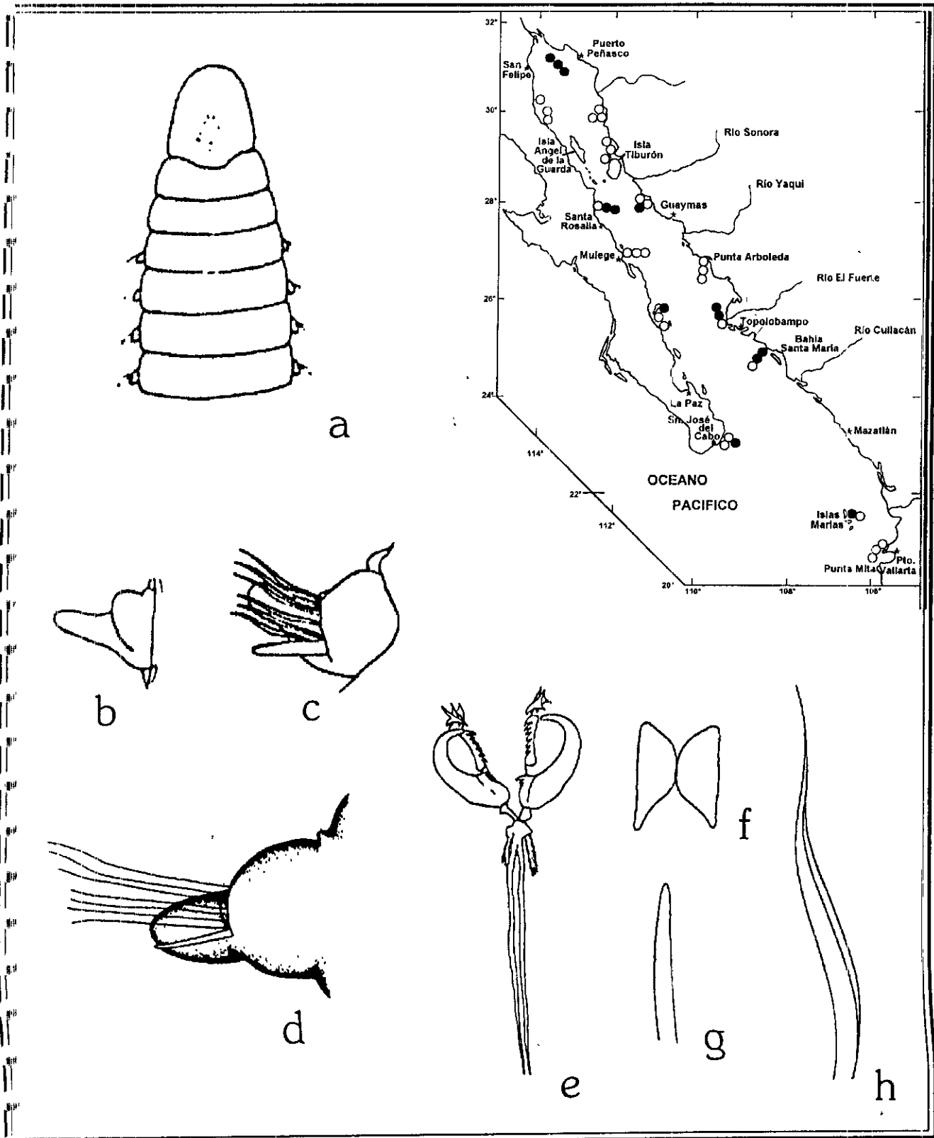
Figura 20.2. Drilonereis falcata : a) Región anterior, vista dorsal; b) Neuropodio anterior; c) Parapodio posterior; d) Parapodio medio; e) Maxilas; f) Mandíbulas; g) Seta limbada; h) Acicula, región distal. Figs. a, f, h: tomadas de Day 1967; b, c, e, g: tomadas de Moore 1911; Fig. d: tomada Fauchald 1970.
