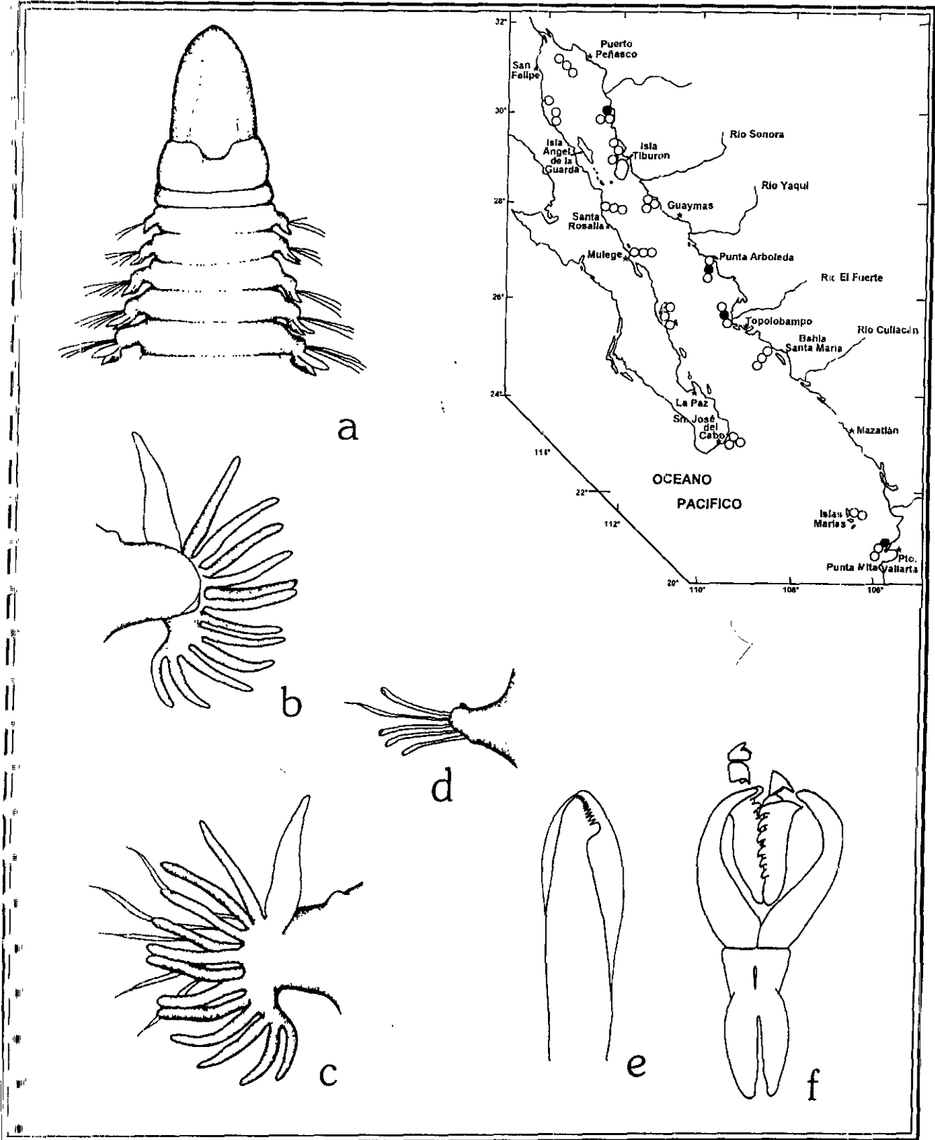
Figura 19.3. Ninoe foliosa : a) Región anterior, vista dorsal; b) Parapodio 19, vista anterior setas omitidas; c) Parapodio 19, vista posterior; d) Parapodio posterior; e) Gancho simple, setífero posterior; f) Maxila. Figs. Tomadas de Fauchald 1972a.
