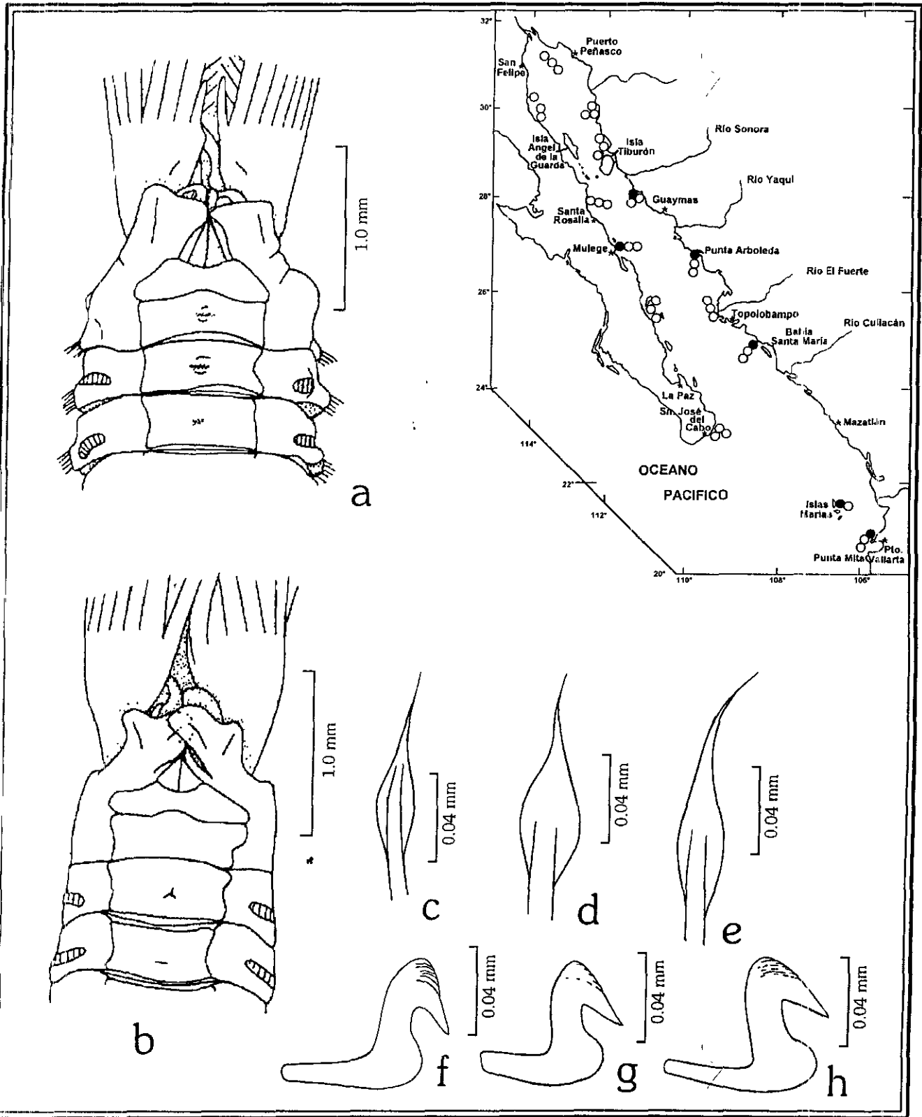
Figura 40.4. Megalomma pigmentum : a) Región anterior y parte de la corona branquial, vista ventral; b) Región anterior, otro organismo; c, d) Setas superiores; e) Seta inferior; f-h) Ganchos torácicos aviculares. Figs. Tomadas de Perkins 1984.
