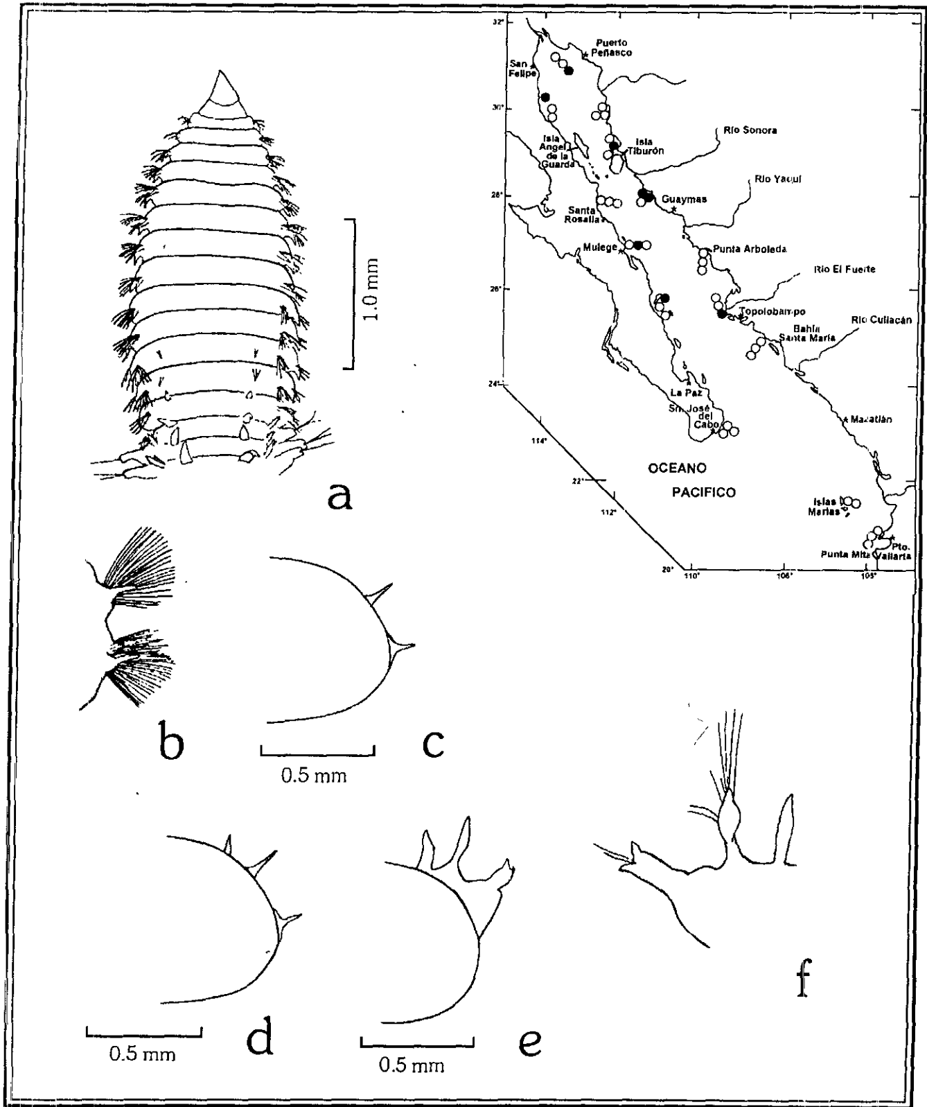
Figura 22.1. Leitoscoloplos mexicanus : a) Región anterior, vista dorsal; b) Octavo parapodio; c-e) Setígeros 9, 10 y 16, sin setas; f) Parapodio abdominal. Figs. a, c-e: tomadas de Mackie 1987; Figs. b,f: tomadas de Fauchald 1972a
