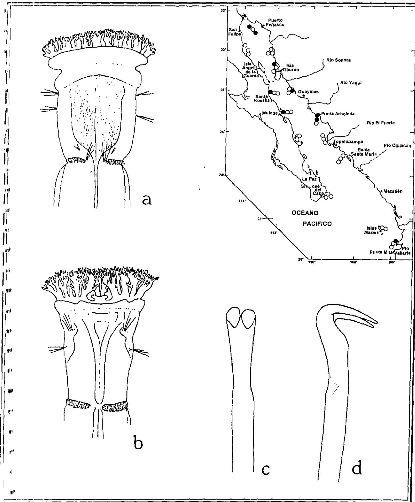
Figura 36.1. Owenia collaris : a) Región anterior, vista dorsal; b) Región anterior, vista ventral; c) Uncino con dos dientes largos, vista frontal; d) El mismo, vista lateral. Figs. Tomadas de Hartman 955. 1969.
