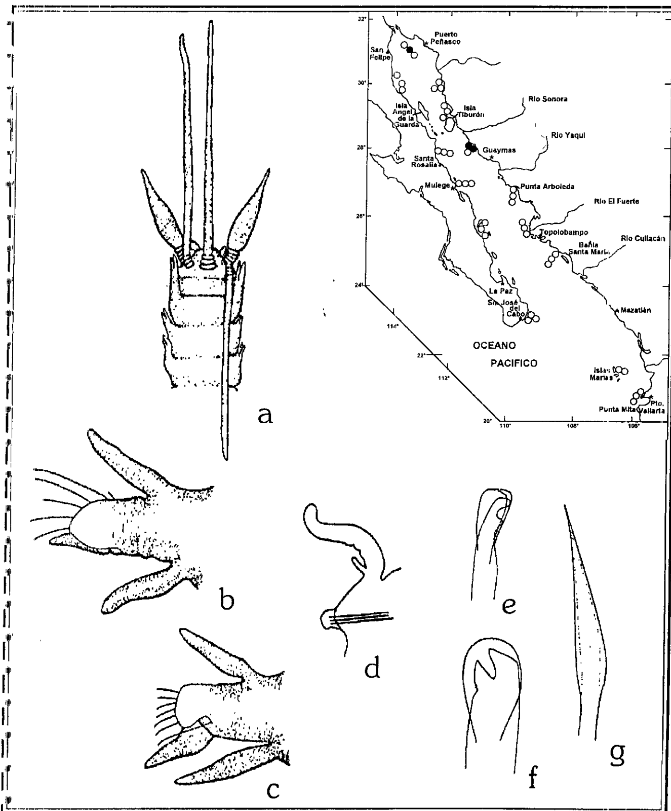
Figura 17.7. Hyalinoecia juvenalis : a) Región anterior, vista dorsal; b, c) Primer setígero; d) Setígero 25; e) Gancho cubierto del segundo parapodio; f) Gancho subacicular, parapodio 30; g) Seta limbada simple. Figs. a-c, e, f: tomadas de Fauchald 1968; Figs. d, g: tomadas de Moore 1911.
