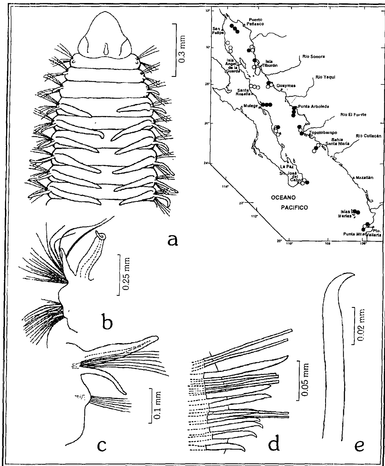
Figura 23.4. Aricidea (Acmira) simplex : a) Región anterior, vista dorsal; b) Parapodio del segmento 8; c) Parapodio del setígero 12; d) Neuropodio posterior; e) Neuroseta modificada. Figs. a, c, e: tomadas de Gaston 1984; Figs. b, d: tomadas de Strelzov 1979.
