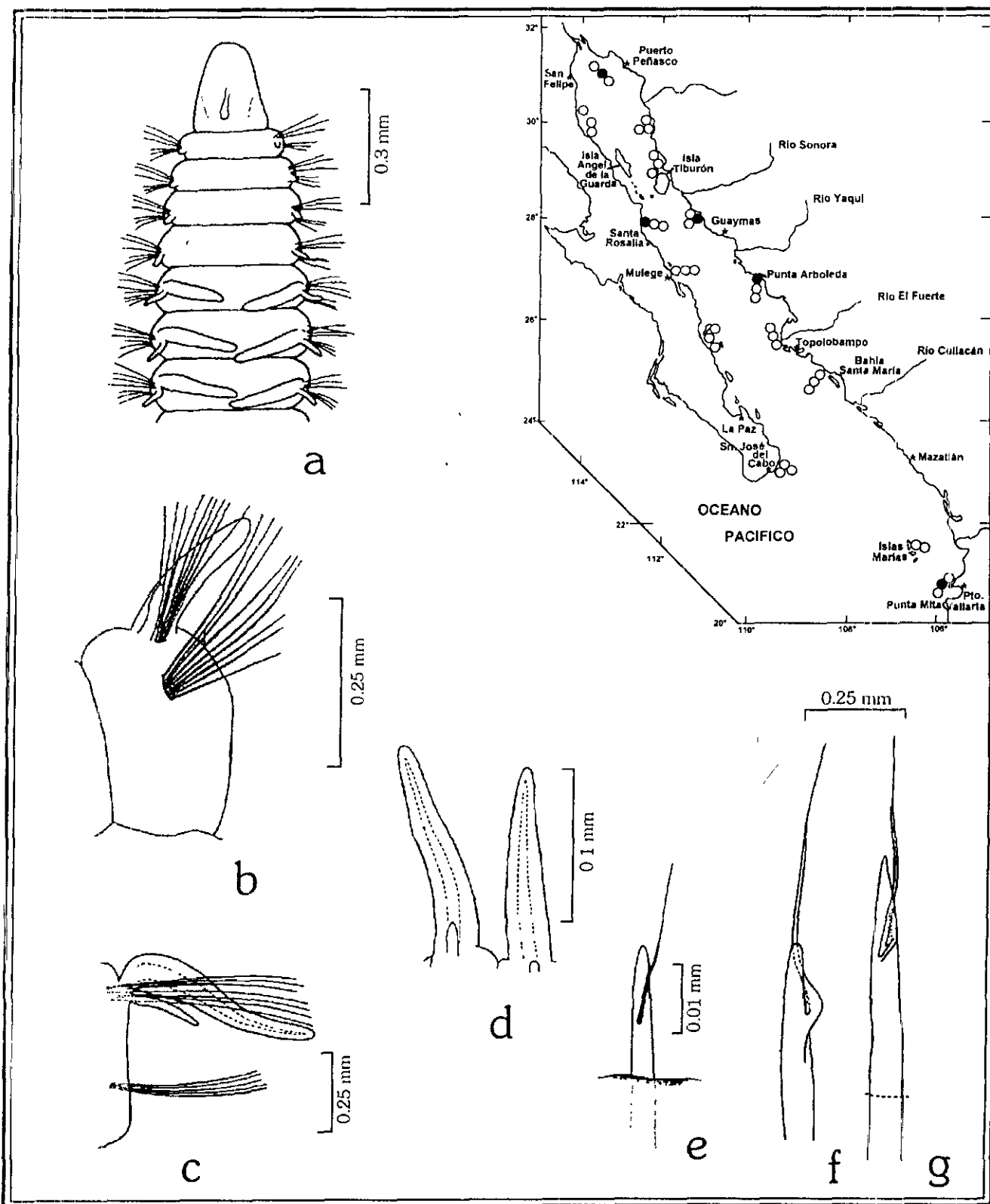
Figura 23.8. Cirrophorus branchiatus : a) Región anterior, vista dorsal; b) Sexto segmento, vista lateral; c) Setígero 10; d) Branquias; e-g) Setas modificadas. Figs. a, c, e: tomadas de Gaston 1984.; Figs. b, d, f, g: tomadas de Strelzov 1979.
