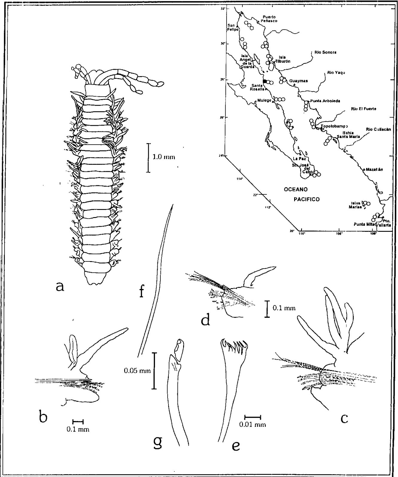
Figura 18.1. Eunice mexicana : a) Organismo completo, vista dorsal; b) Setígero 3; c) Setígero 10; d) Setígero 24; e) Seta pectinada; f) Seta limbada; g) Gancho bidentado, vista lateral.
