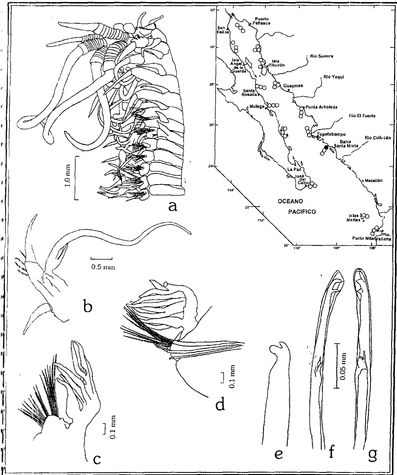
Figura 17.6. Hirsutonuphis acapulcensis : a) Región anterior, vista lateral; b) Setígero 5; c) Setígero 15; d) Setígero 20; e) Gancho pseudocompuesto del setígero 5; f) Gancho subacicular del setígero 20.
