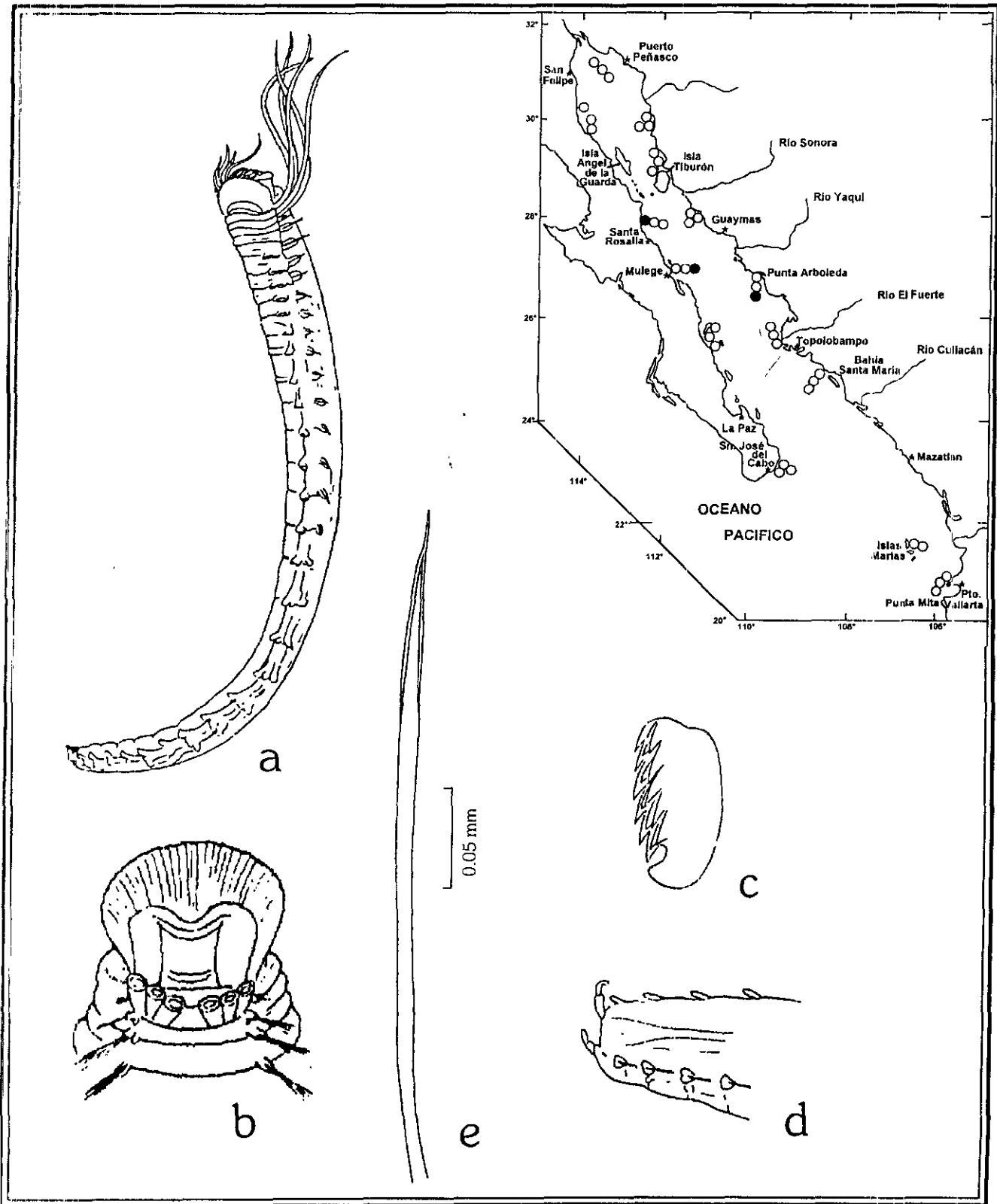
Figura 37.7. Samytha sexcirrata : a) Organismos completo, vista lateral; b) Región anterior con branquias; c) Uncino con dientes en líneas múltiples; d) Región posterior, vista dorsal; e) Seta del parapodio 4. Figs. a-d: tomadas de Wollebaek 1912.
