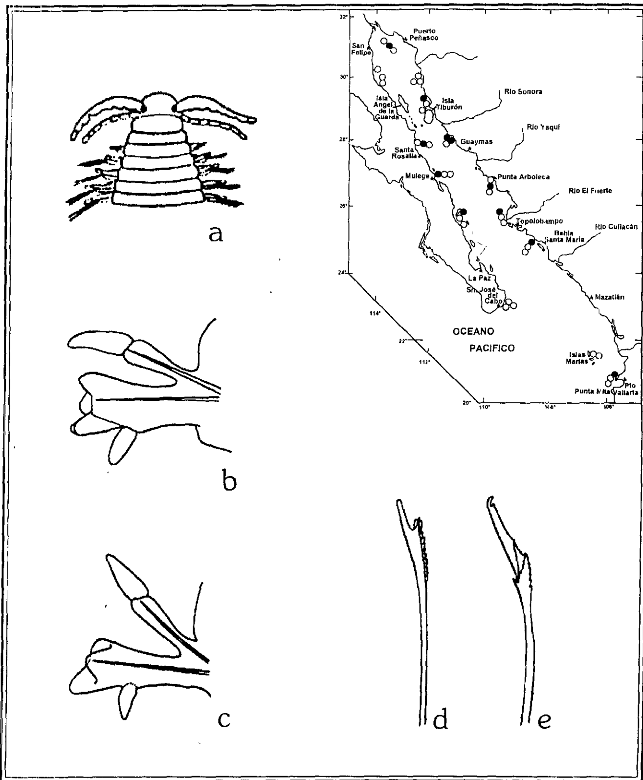
Figura 21.2. Schistomeringos longicornis : a) Región anterior, vista dorsal; b) Parapodio medio; c) Parapodio posterior; d) Seta superior simple; e) Seta inferior compuesta. Fig. a: tomada de Fauvel 1923; Figs. b-e: tomadas de Hartman 1938.
