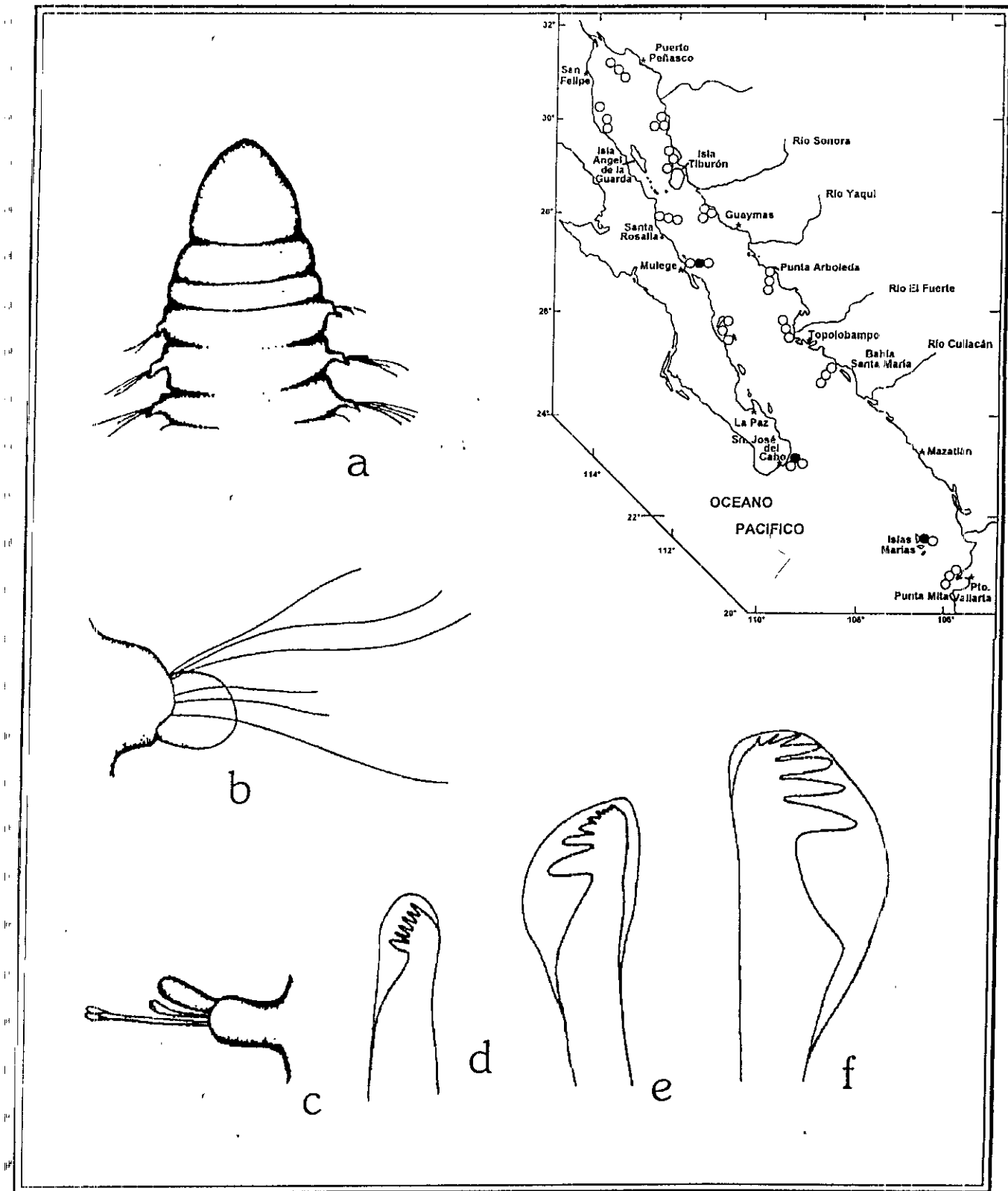
Figura 19.5. Lumbrineris crassidentata : a) Región anterior, vista dorsal; b) Parapodio 2; c) Parapodio posterior; d) Gancho cubierto simple, segundo setífero; e) Gancho cubierto simple, setífero 200; f) Gancho cubierto simple, setífero 100. Figs. Tomadas de Fauchald 1970.
