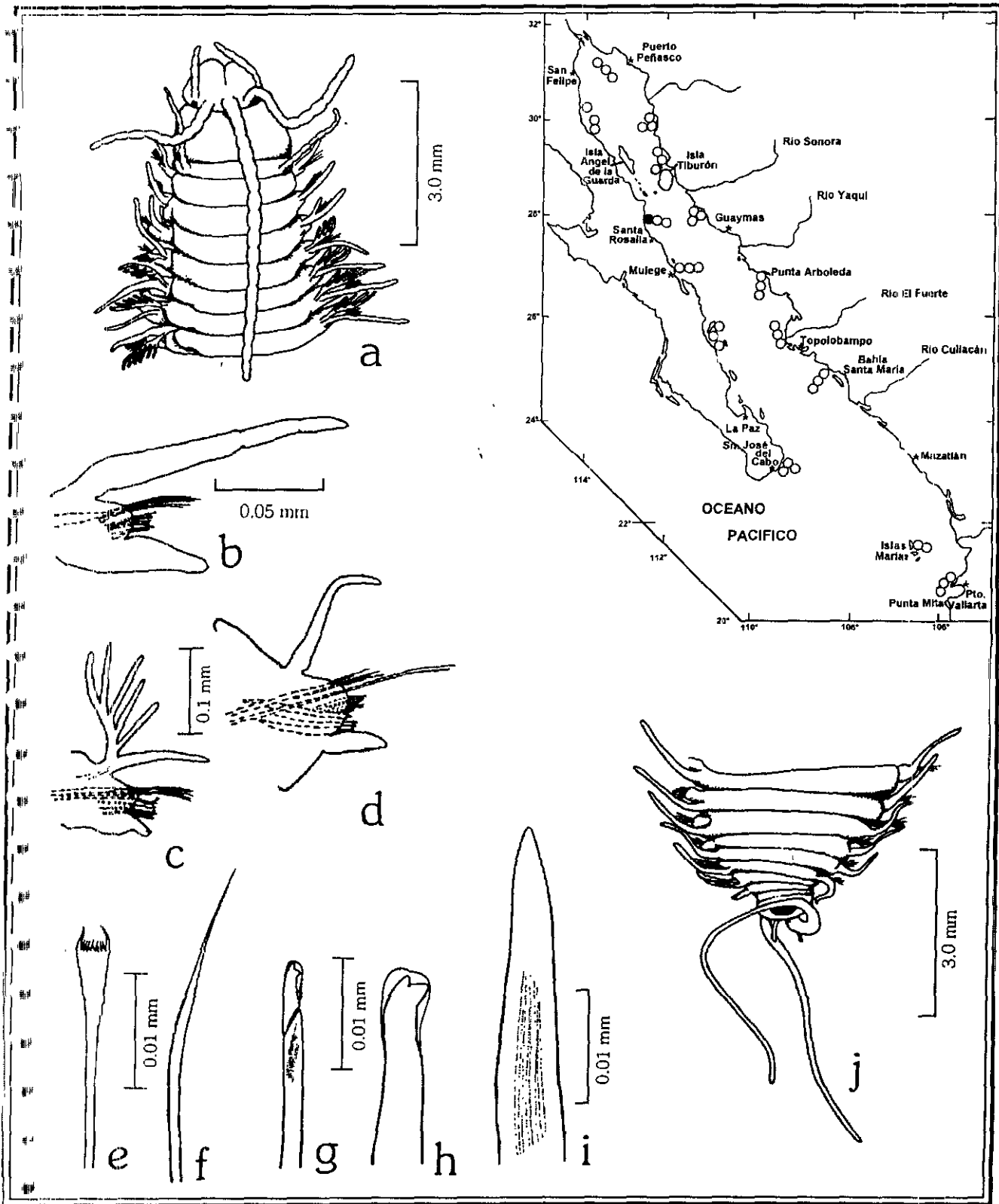
Figura 18.3. Eunice websteri : a) Región anterior, vista dorsal; b) Parapodio anterior; c) Parapodio branquial; d) Parapodio posterior; e) Seta pectinada; f) Seta limbada; g) Falcigero compuesto; h) Gancho cubierto subacicular; i) Acicula; j) Región posterior, vista dorsal. Figs. Tomadas de Gathof 1984.
