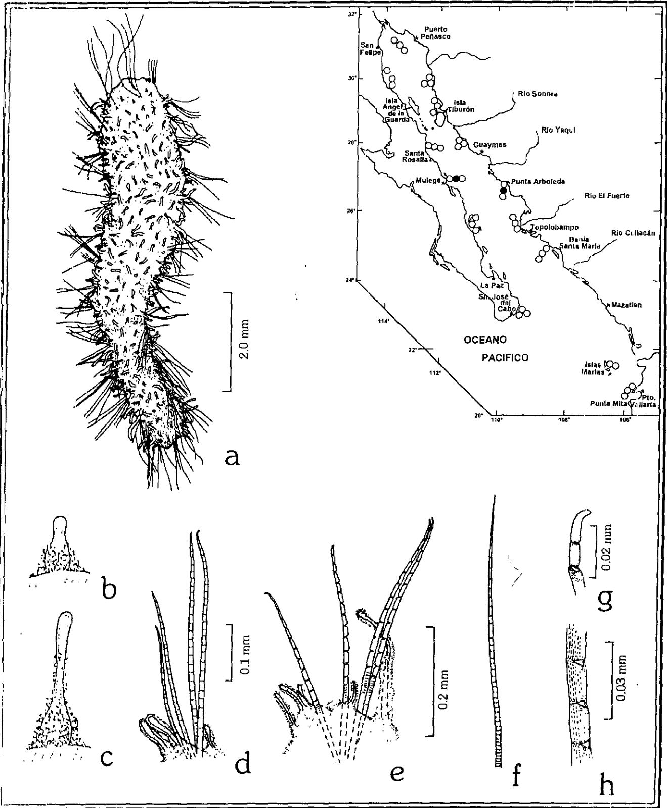
Figura 3.1.2. Diplocirrus capensis : a) Organismo completo, vista dorsal; b) Papila de la superficie ventral; c) Papila de la superficie dorsal; d) Notopodio del setígero 6; e) Neuropodio del setígero 6; Notoseta; g) Neuroseta de la región distal; h) Notoseta. Figs. a, d, e, g, h: tomadas de Milligan 1984; b, c, f: tomadas de Day 1967.
