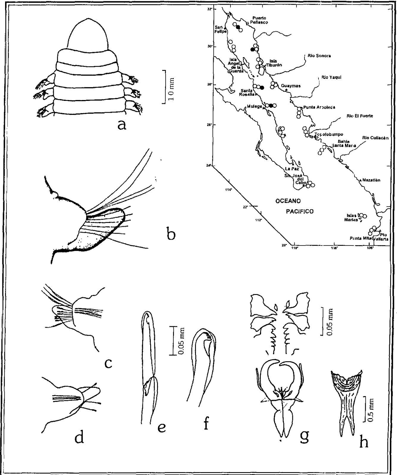
Figura 19.8. Lumbrineris latreilli : a) Región anterior, vista dorsal; b) Parapodio 5; c) Parapodio anterior; d) Parapodio posterior; e) Gancho compuesto cubierto de un parapodio anterior; f) Gancho cubierto de un parapodio posterior; g) Maxila; h) Mandibula. Figs. a, e-h: tomadas de Orenzans 1973; Figs. c, d: tomadas de Gardiner 1976; Fig. b: tomada de Fauchald 1970.
