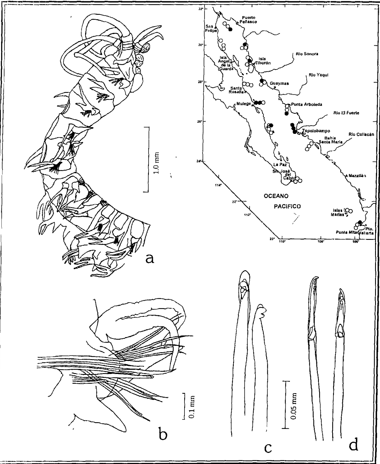
Figura 17.8. Kinbergonuphis cedroensis : a) Región anterior, vista lateral; b) Setígero 6; c) Gancho tridentado pseudocompuesto del setígero 4; d) Ganchos simples del setígero 6.
